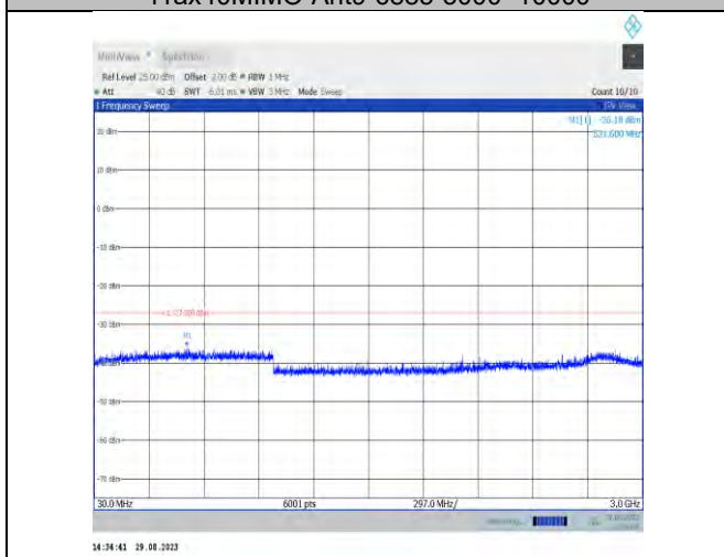
11ax40MIMO-Ant7-6925-30~3000
