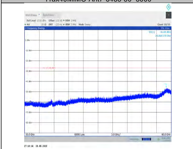
11ax40MIMO-Ant7-6485-10000~40000
