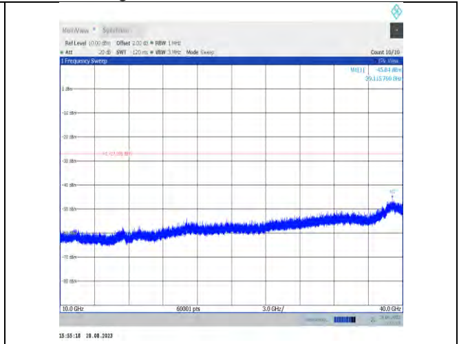
11ax20MIMO-Ant9-7115-10000~40000
