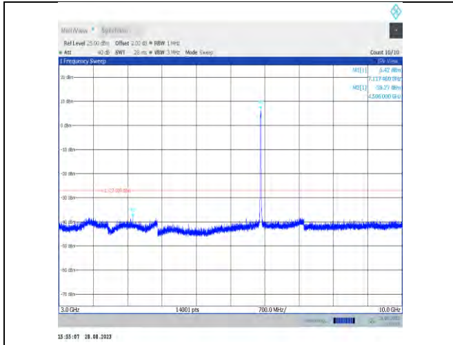
11ax20MIMO-Ant9-7115-3000~10000
