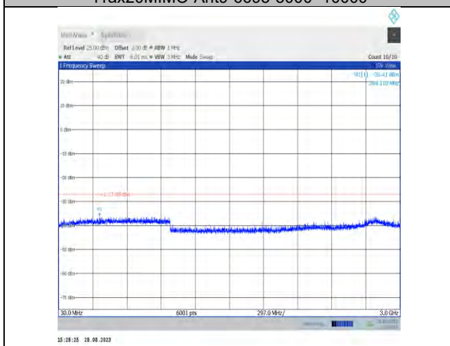
11ax20MIMO-Ant7-6855-30~3000
