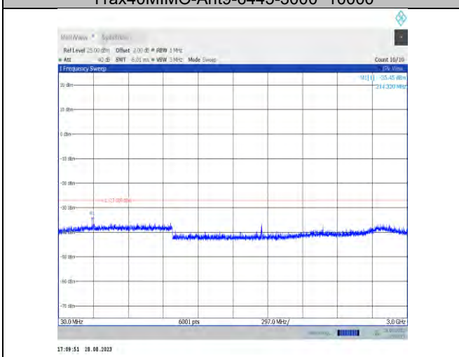
11ax40MIMO-Ant7-6485-30~3000
