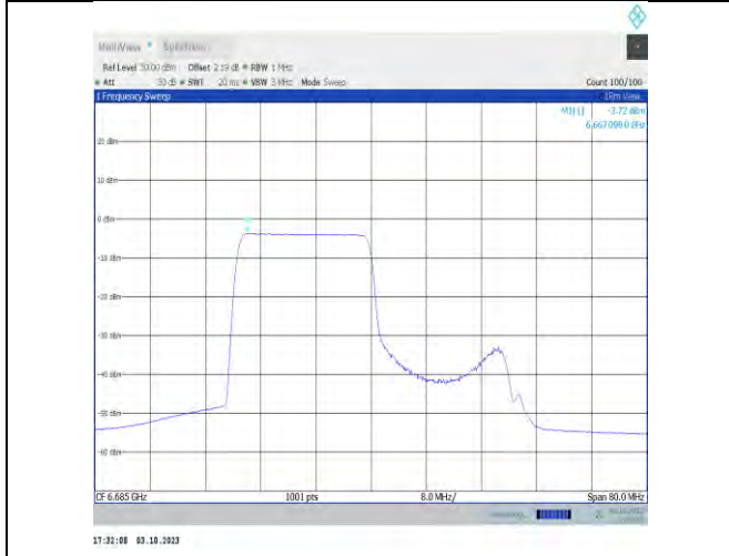
11x40MIMO-Ant7-6685-PASS
