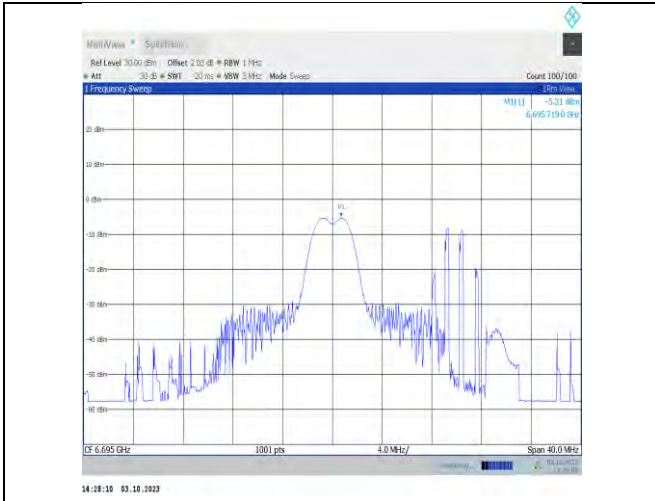
11ax20MIMO-Ant7-6695-PASS
