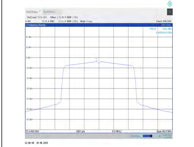
11ax40MIMO-Ant7-6685-PASS
