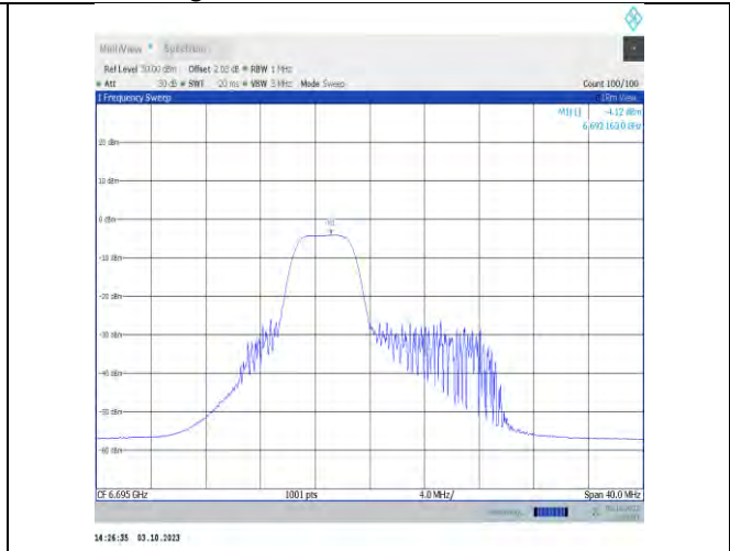
11ax20MIMO-Ant7-6695-PASS
