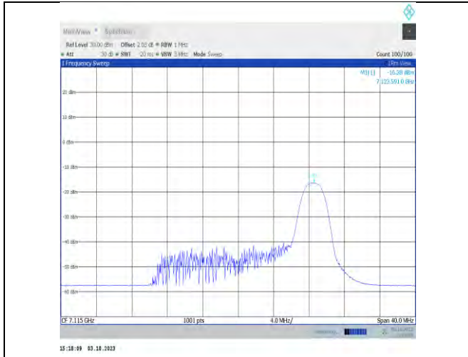
11ax20MIMO-Ant7-7115-PASS
