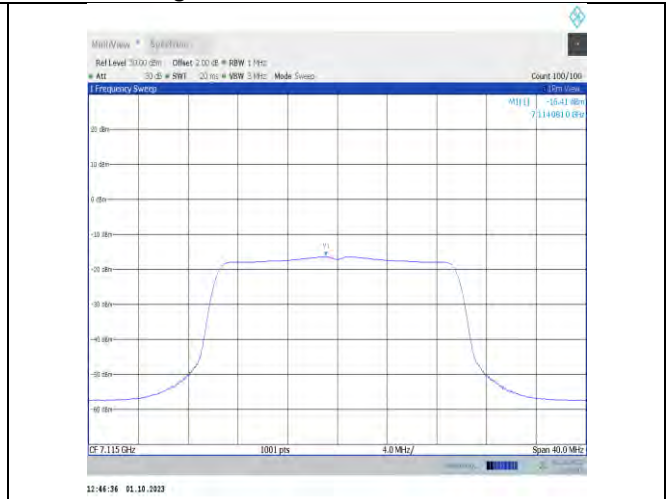
11x20MIMO-Ant9-7115-PASS
