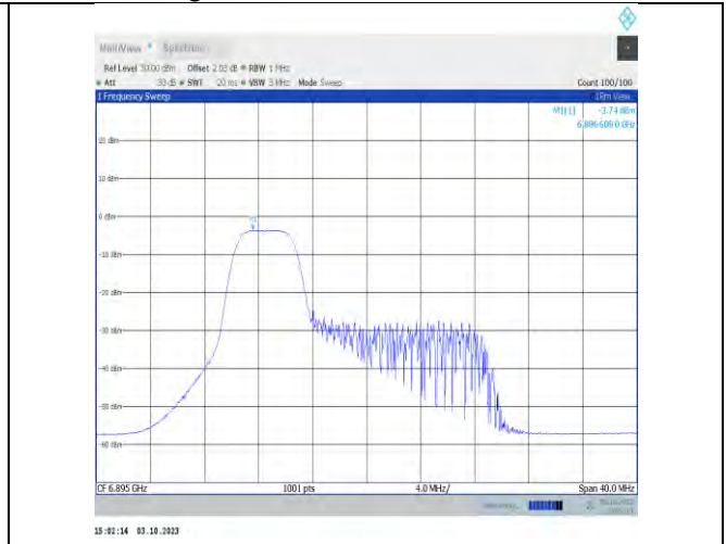
11x20MIMO-Ant7-6895-PASS
