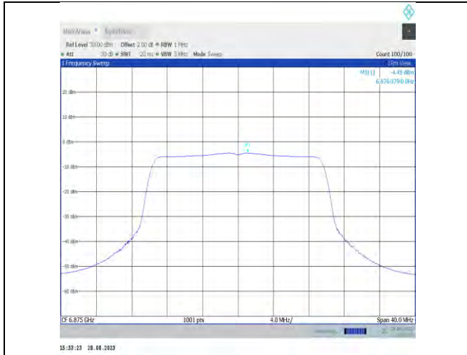
11x20MIMO-Ant7-6875-PASS
