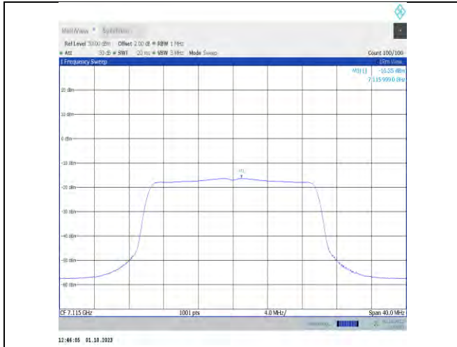
11x20MIMO-Ant7-7115-PASS
