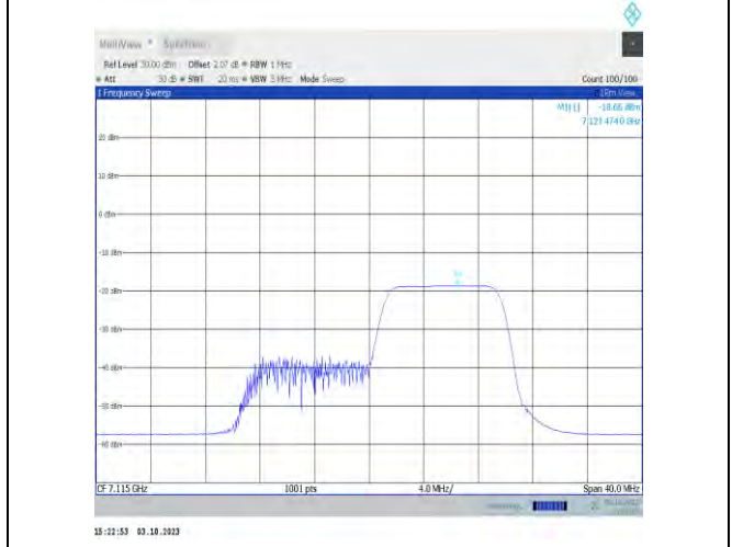
11ax20MIMO-Ant9-7115-PASS
