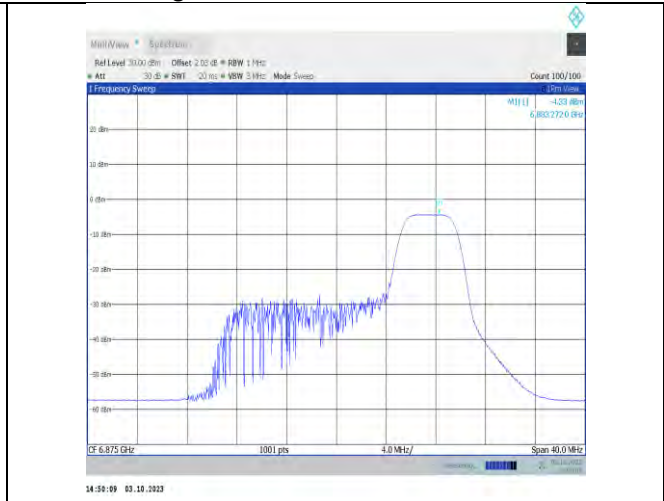
11ax20MIMO-Ant7-6875-PASS
