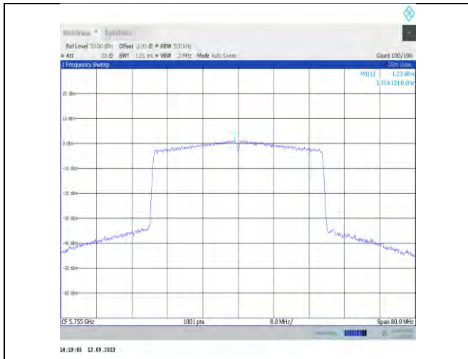
11ax40MIMO-Ant7-5755-PASS
