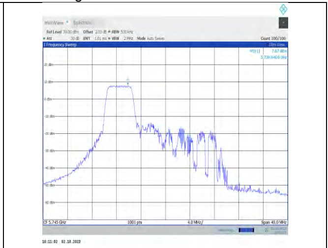
11ax20MIMO-Ant7-5745-PASS
