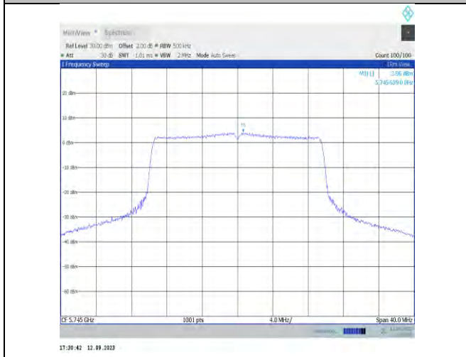
11ax20MIMO-Ant7-5745-PASS
