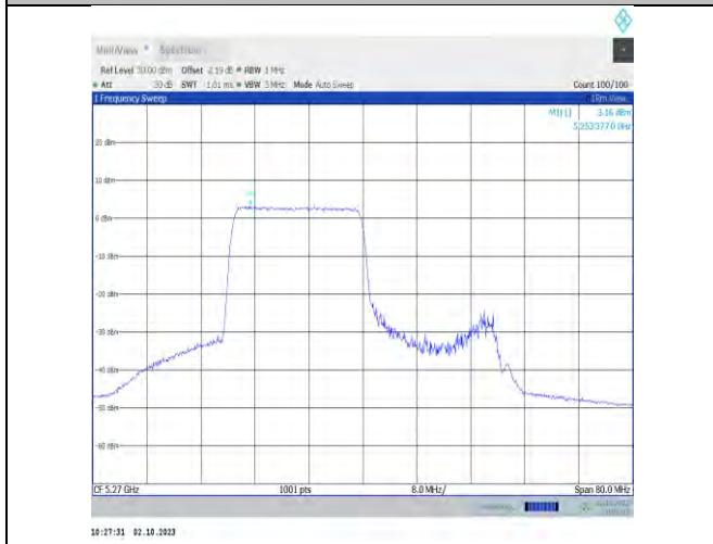
11ax40MIMO-Ant7-5270-PASS
