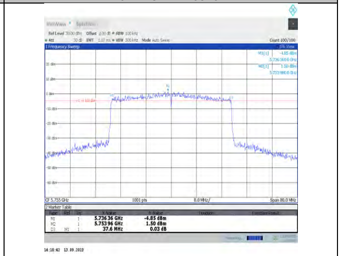
11ax40MIMO-Ant7-5755-PASS
