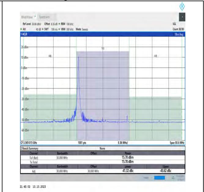
NTVN_N48_PC3_30_30_L_TID2_#1_-30_30
