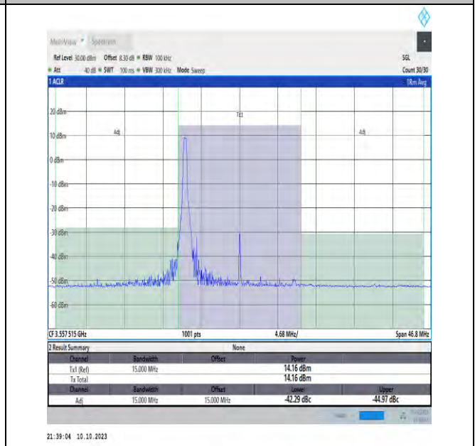
NTVN_N48_PC3_30_15_L_TID17_#1_-15_15
