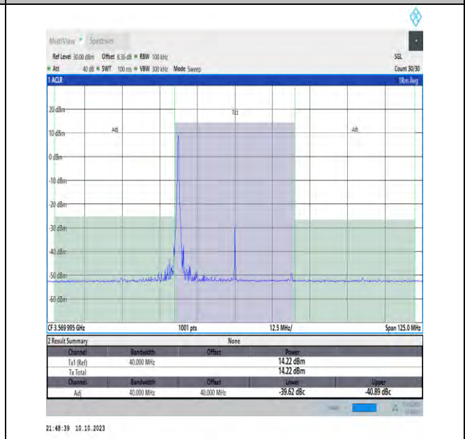
NTVN_N48_PC3_30_40_L_TID17_#1_-40_40
