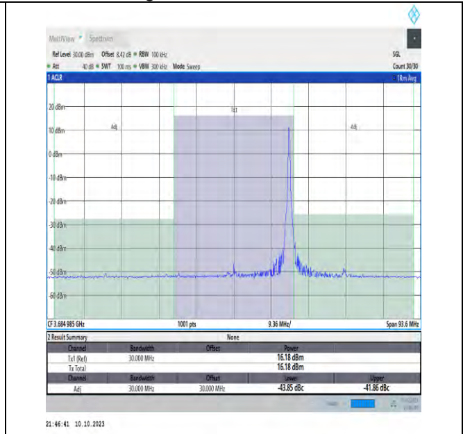
NTVN_N48_PC3_30_30_H_TID3_#1_-30_30
