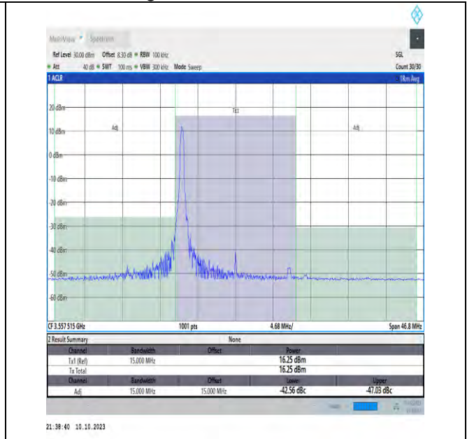
NTVN_N48_PC3_30_15_L_TID2_#1_-15_15
