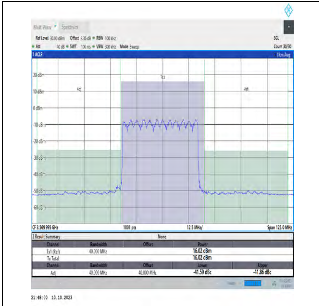
NTVN_N48_PC3_30_40_L_TID1_#1_-40_40
