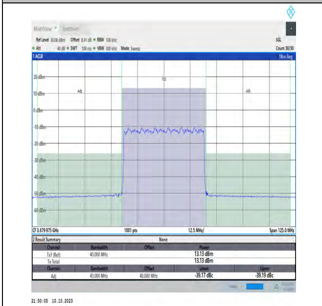
NTVN_N48_PC3_30_40_H_TID16_#1_-40_40
