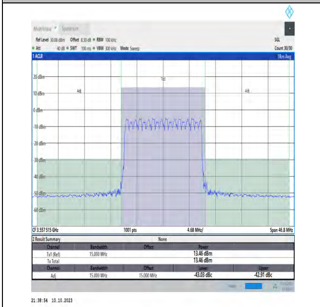
NTVN_N48_PC3_30_15_L_TID16_#1_-15_15
