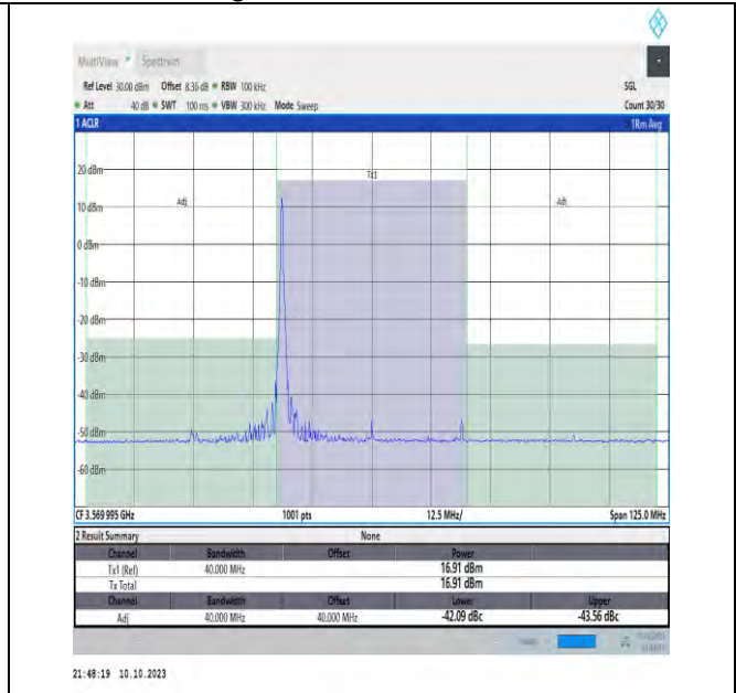
NTVN_N48_PC3_30_40_L_TID2_#1_-40_40
