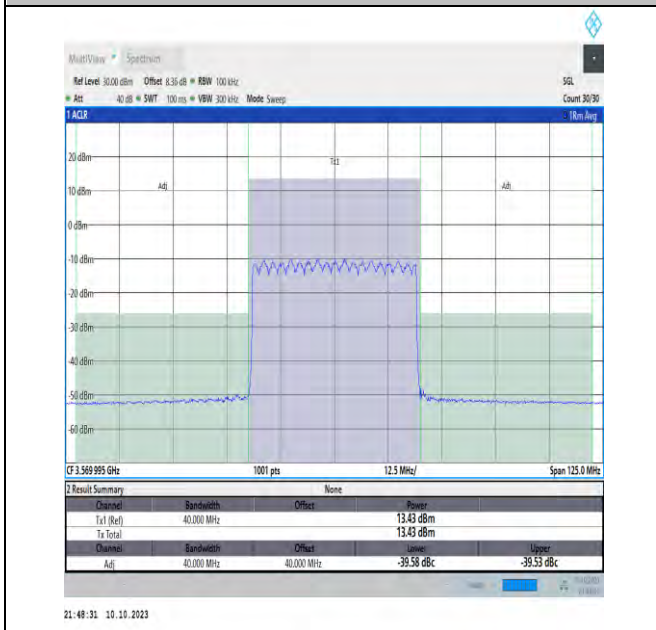
NTVN_N48_PC3_30_40_L_TID16_#1_-40_40
