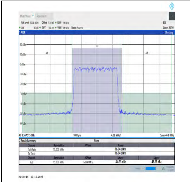
NTVN_N48_PC3_30_15_L_TID1_#1_-15_15
