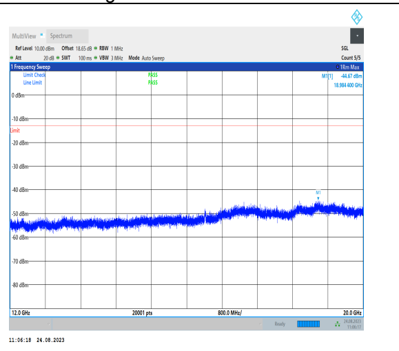
1-N71-PC3-15-20-H-1-DFT-PI2BPSK-Inner_1RB_Lef t-1@1-12000-20000-Ant1-18984.40--44.67--13-PASS
