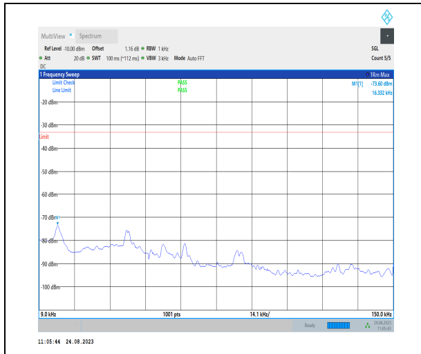
1-N71-PC3-15-20-H-1-DFT-PI2BPSK-Inner_1RB_L eft-1@1-0.009-0.15-Ant1-0.02--73.60--33-PASS
