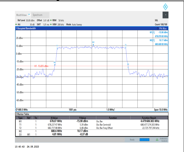
1-N71-PC3-15-5-M-6-CP-QPSK-Outer_Full-25@0-A nt1-4.48-4.810-≤5-PASS
