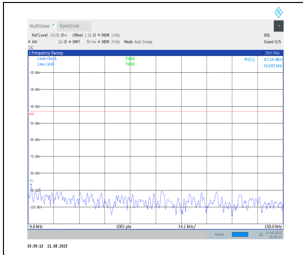
1-N66-PC3-15-40-H-1-DFT-PI2BPSK-Inner_1RB_L eft-1@1-0.009-0.15-Ant3-0.01--87.58--43-PASS
