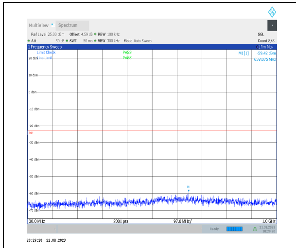
1-N66-PC3-15-40-M-1-DFT-PI2BPSK-Inner_1RB_L eft-1@1-30-1000-Ant3-658.08--59.42--23-PASS
