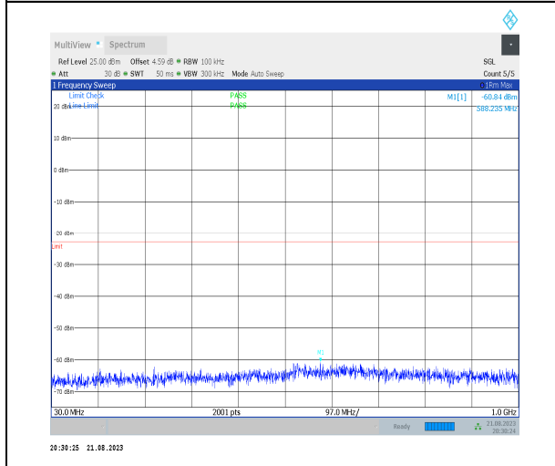
1-N66-PC3-15-40-H-1-DFT-PI2BPSK-Inner_1RB_L eft-1@1-30-1000-Ant3-588.24--60.84--23-PASS
