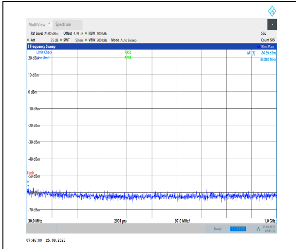
1-N30-PC3-15-10-M-1-DFT-PI2BPSK-Inner_1RB_L eft-1@1-30-1000-Ant3-33.88--56.89--50-PASS
