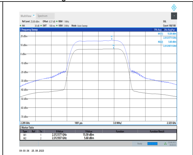
1-N30-PC3-15-10-H-2-CP-256QAM-Outer_Full-52@ 0-Ant3-9.99-100%-0.00-9.99-PASS-≤13
