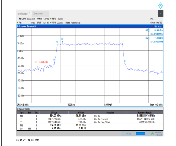
1-N26-824-849-PC3-15-5-M-7-CP-16QAM-Outer_Full-25@0-Ant1-4.467-4.810-≤5-PASS
