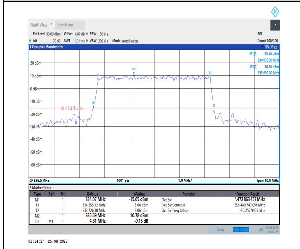
1-N5-PC3-15-5-M-7-CP-16QAM-Outer_Full-25@0-A nt1-4.473-4.810-≤5-PASS
