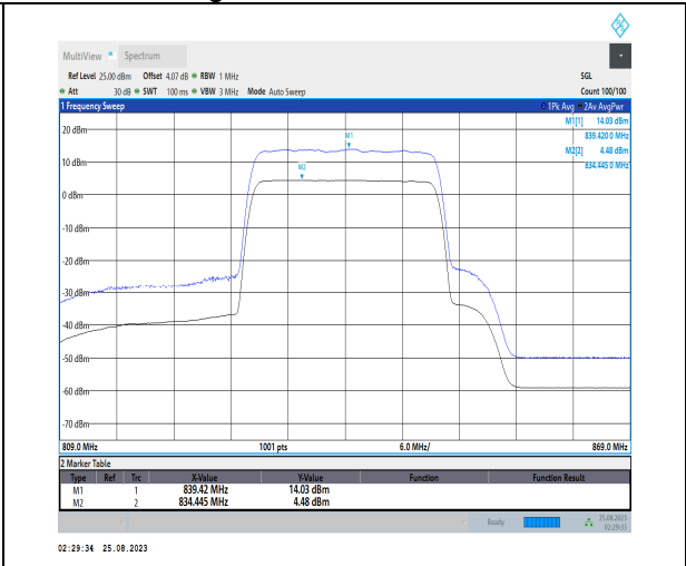
1-N5-PC3-15-20-H-2-CP-256QAM-Outer_Full-106@ 0-Ant1-9.55-100%-0.00-9.55-PASS-≤13
