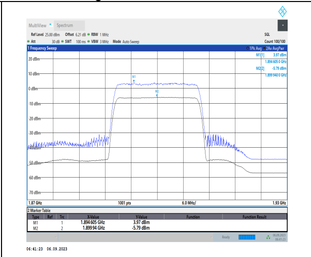
1-N2-PC3-15-20-H-2-CP-256QAM-Outer_Full-106@ 0-Ant3-9.76-100%-0.00-9.76-PASS-≤13
