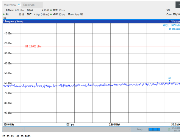
Band14-10MHz-QPSK-23330-1RB#0-Range2:0.15~30MHz
