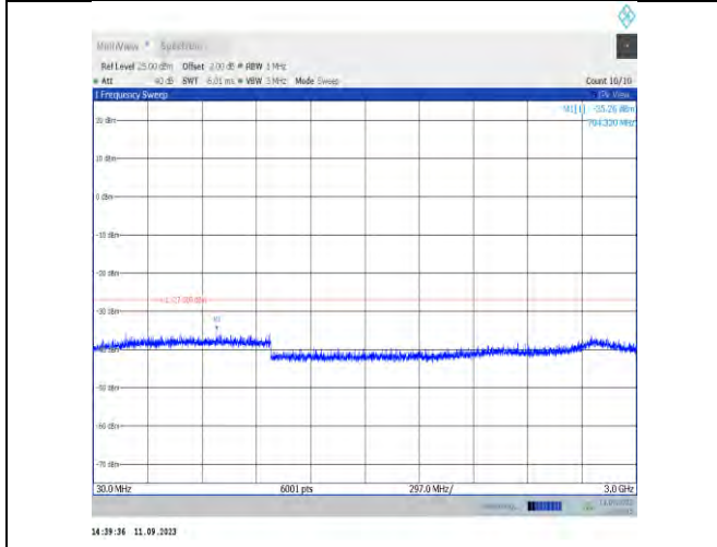
11ax40MIMO-Ant7-6525-30~3000
