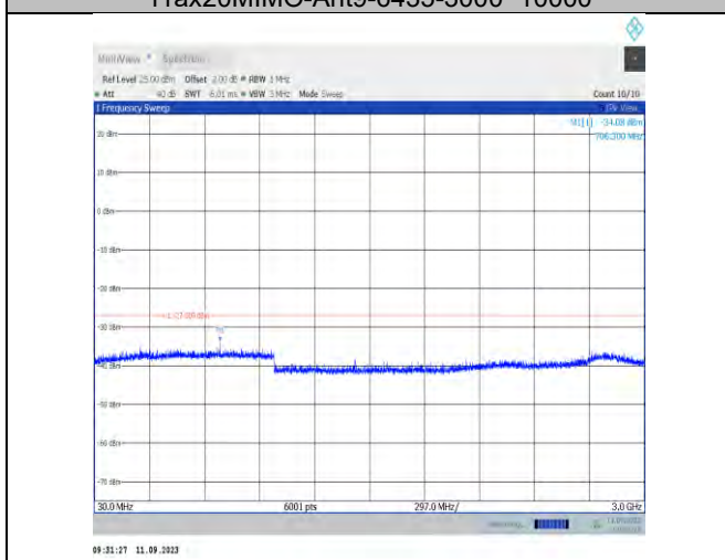
11ax20MIMO-Ant7-6475-30~3000
