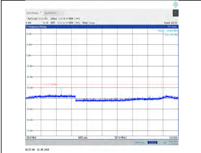
11ax40MIMO-Ant7-6445-30~3000
