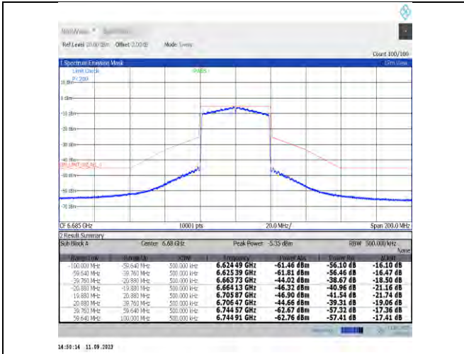
NTNV-11ax40MIMO-Ant7-6685-PASS
