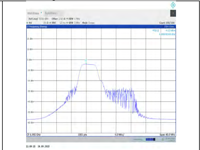
11ax20MIMO-Ant7-6995-PASS
