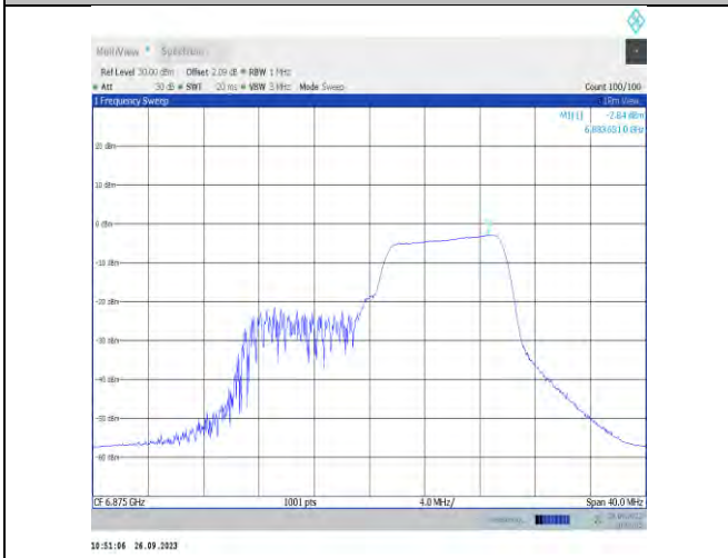
11ax20MIMO-Ant7-6875-PASS
