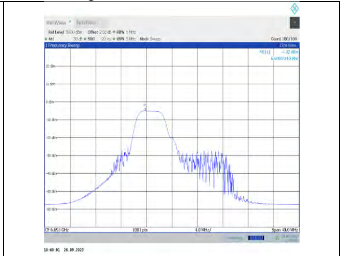
11ax20MIMO-Ant7-6695-PASS
