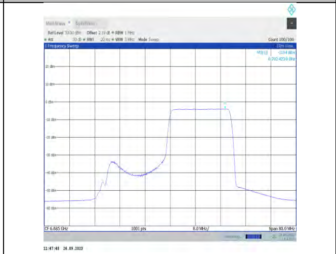
11ax40MIMO-Ant9-6685-PASS
