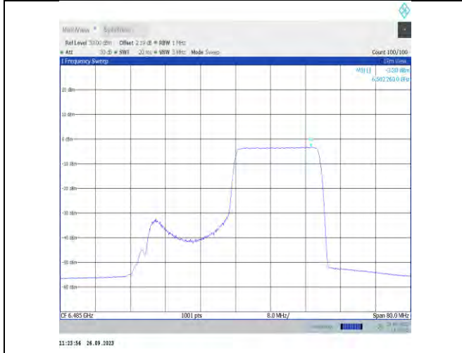
11ax40MIMO-Ant7-6485-PASS
