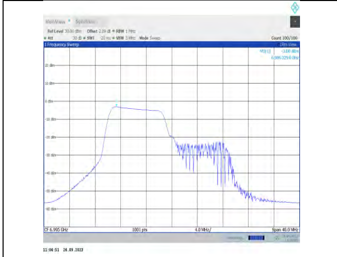
11ax20MIMO-Ant7-6995-PASS
