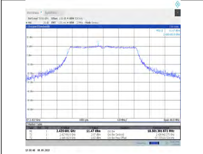
11ax20MIMO-Ant7-2437
