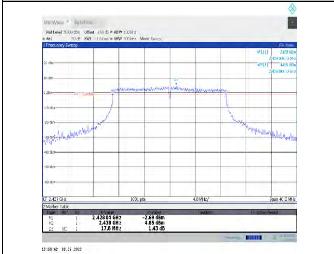
11x20MIMO-Ant7-2437-PASS
