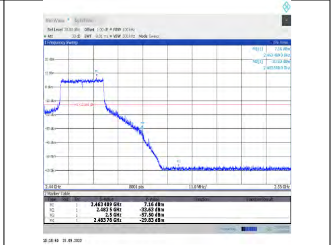
11ax20MIMO-Ant7-2457-PASS
