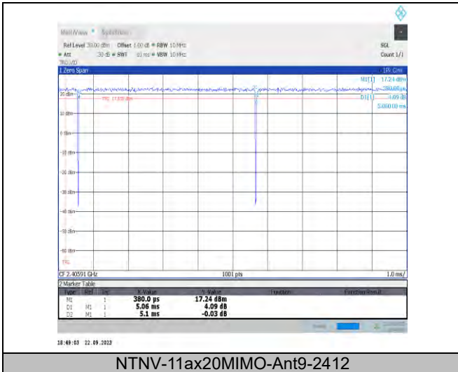
NTNV-11ax20MIMO-Ant9-2412
