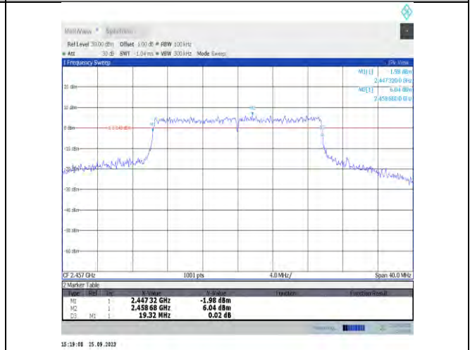
11x20MIMO-Ant9-2457-PASS
