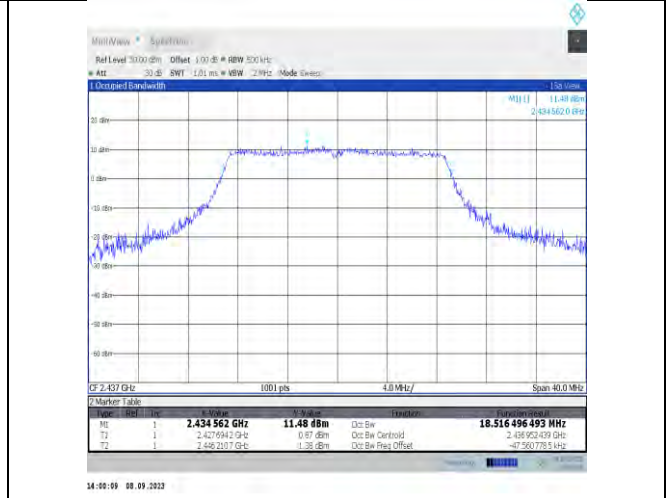
11ax20MIMO-Ant9-2437
