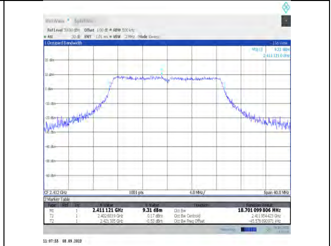
11n20MIMO-Ant9-2412
