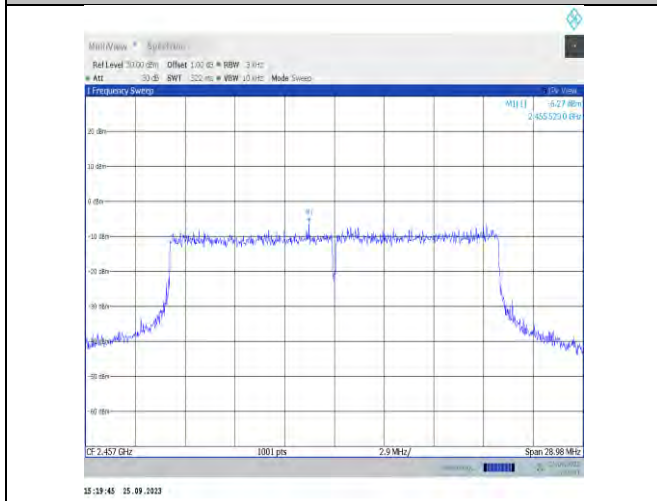
11ax20MIMO-Ant9-2457-PASS
