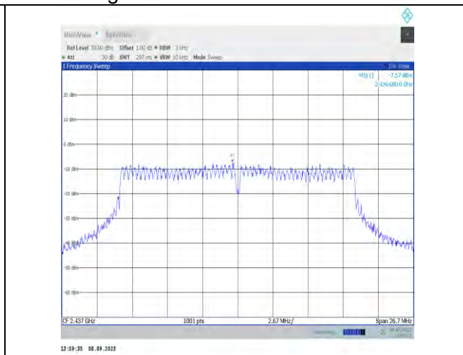
11ax20MIMO-Ant7-2437-PASS
