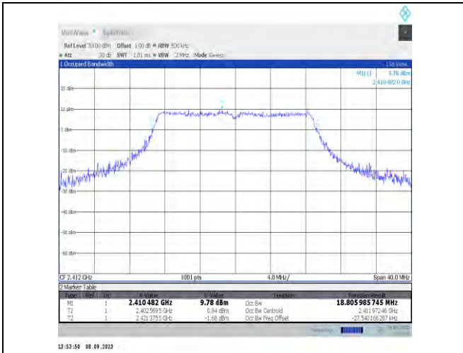
11ax20MIMO-Ant7-2412
