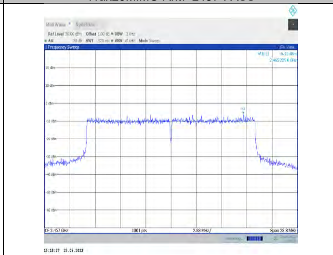
11ax20MIMO-Ant7-2457-PASS
