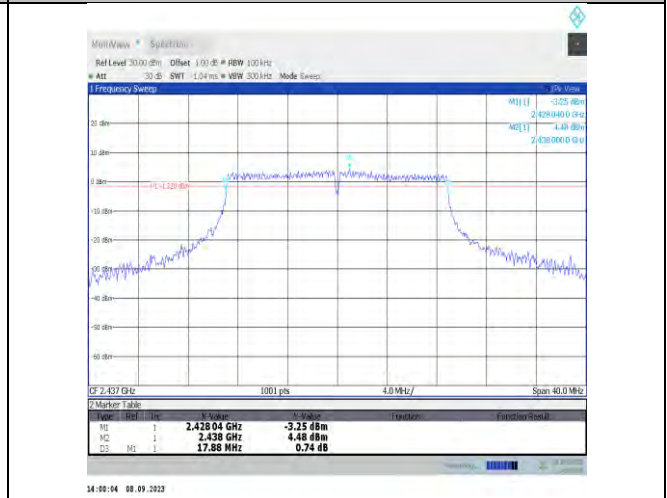
11x20MIMO-Ant9-2437-PASS
