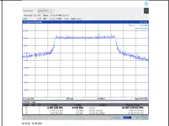
11ax20MIMO-Ant9-2457
