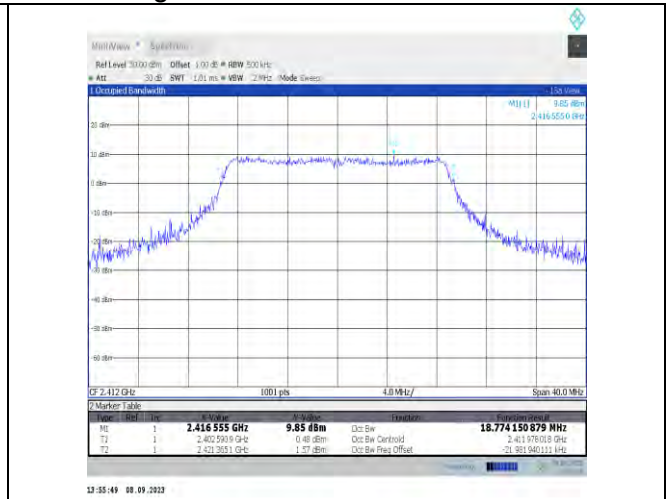
11ax20MIMO-Ant9-2412
