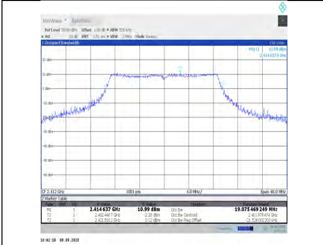
11n20MIMO-Ant7-2412
