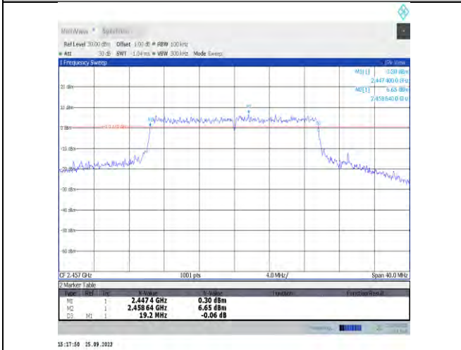
11x20MIMO-Ant7-2457-PASS
