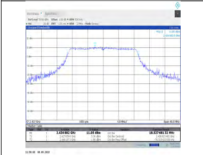
11n20MIMO-Ant7-2437
