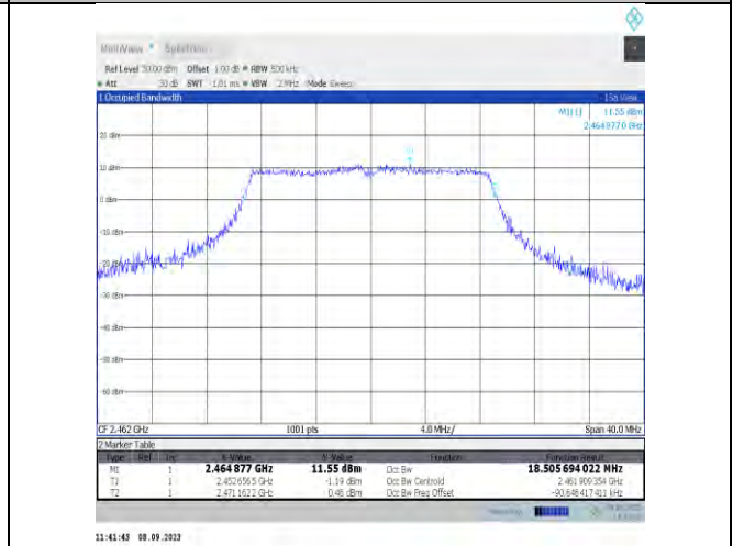
11n20MIMO-Ant9-2462
