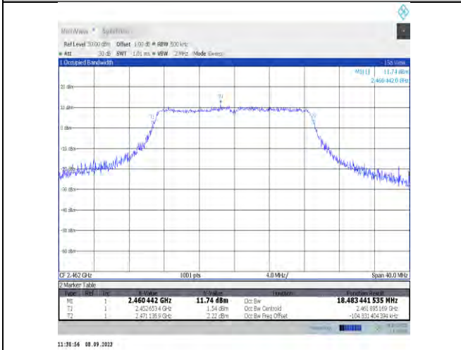
11n20MIMO-Ant7-2462
