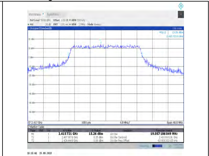
11n20MIMO-Ant9-2417
