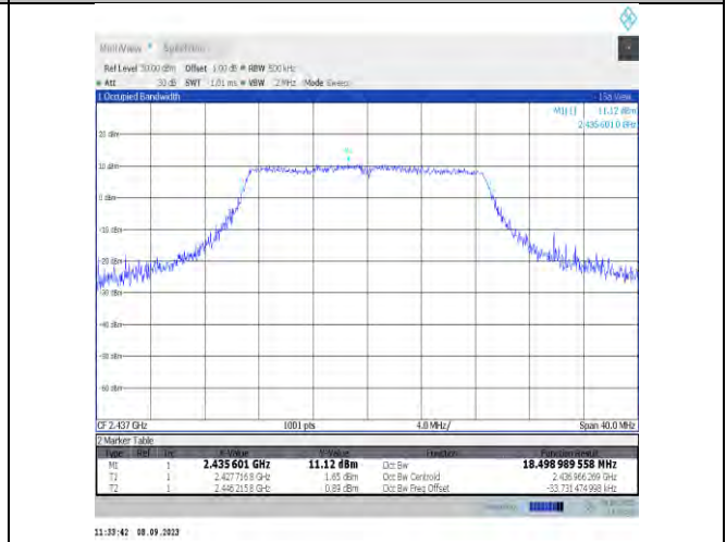
11n20MIMO-Ant9-2437
