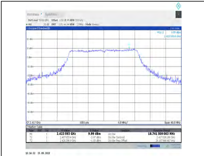
11n20MIMO-Ant7-2417
