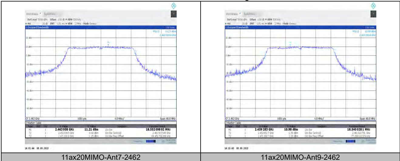
11ax20MIMO-Ant7-2462
