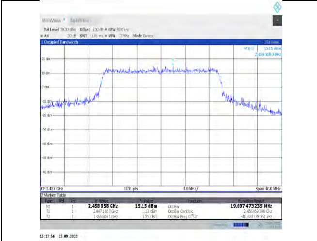
11ax20MIMO-Ant7-2457
