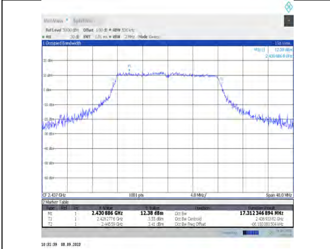
11g-Ant9-2437
