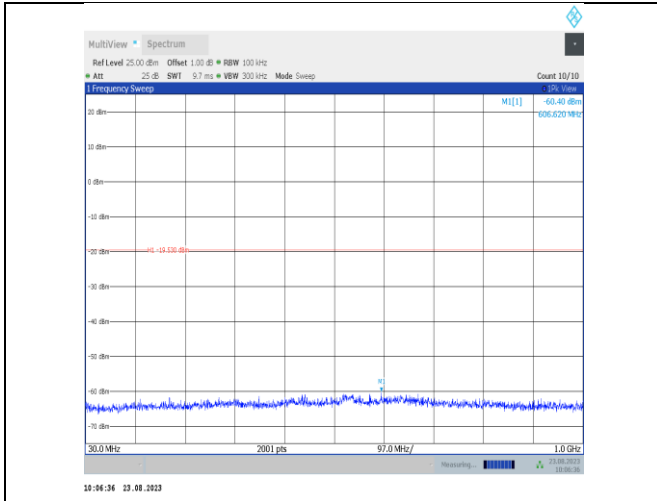
BLE_2M-Ant7-2402-30~1000-PASS
