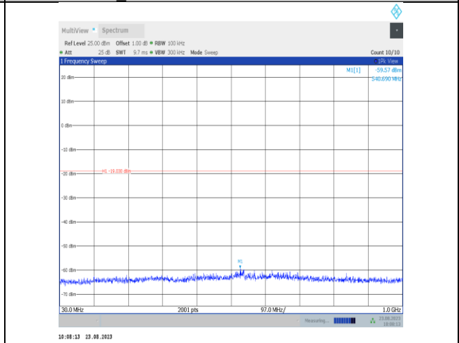
BLE_2M-Ant7-2440-30~1000-PASS
