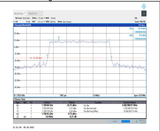
1-N70-PC3-15-5-M-6-CP-QPSK-Outer_Full-25@0-A nt2-4.484-4.800-≤5-PASS
