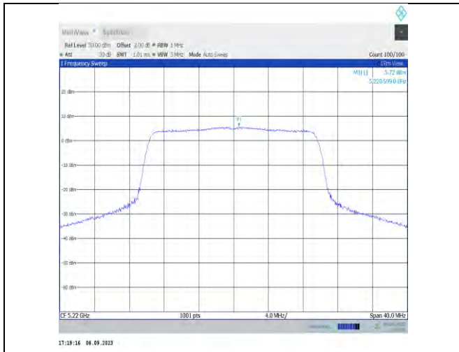
11ax20MIMO-Ant7-5220-PASS
