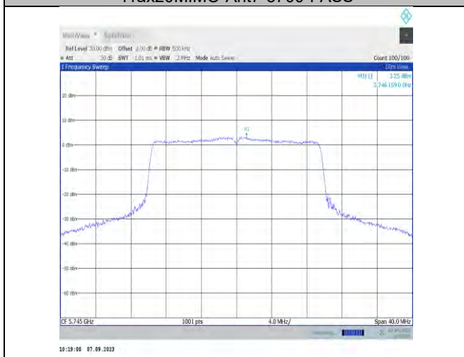
11x20MIMO-Ant7-5745-PASS
