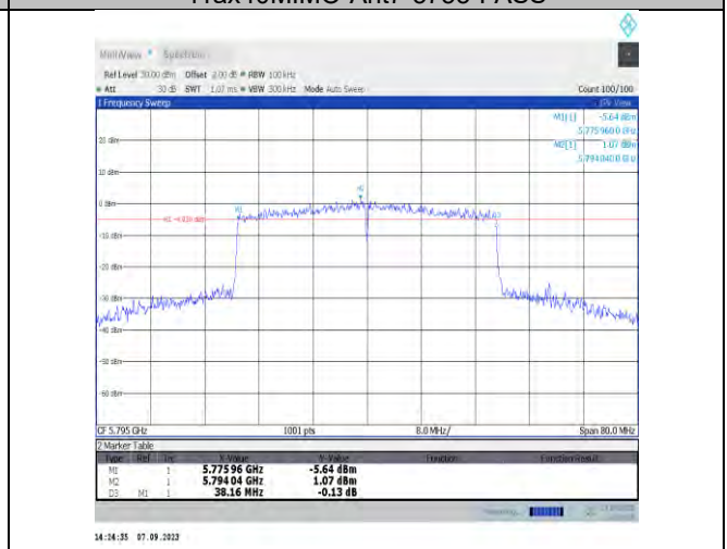
11ax40MIMO-Ant7-5795-PASS
