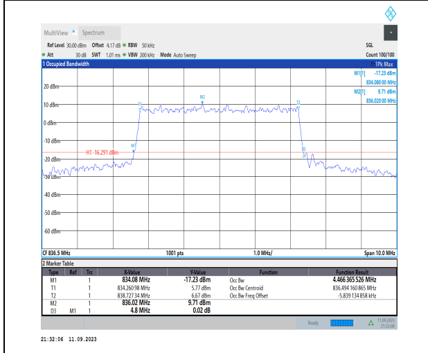
1-N26-824-849-PC3-15-5-M-7-CP-16QAM-Outer_Fu ll-25@0-Ant1-4.466-4.800-≤5-PASS
