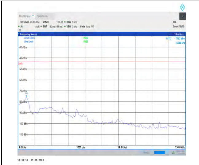
1-N25-PC3-15-40-H-1-DFT-PI2BPSK-Inner_1RB_L eft-1@1-0.009-0.15-Ant2-0.02--75.92--43-PASS
