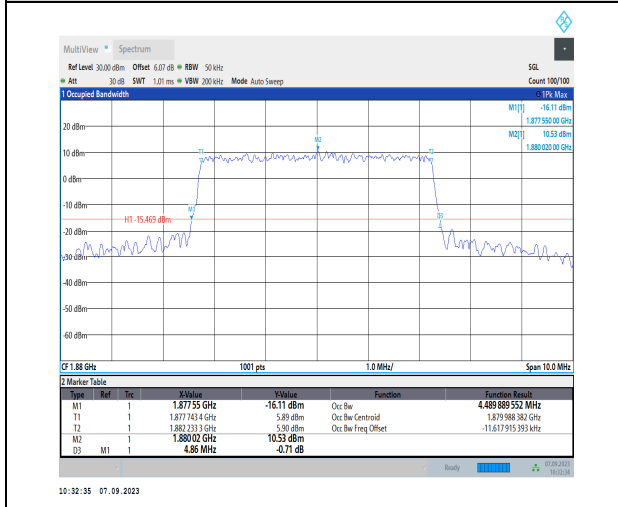
1-N2-PC3-15-5-M-7-CP-16QAM-Outer_Full-25@0-A nt2-4.49-4.860- \leq 5 -PASS
