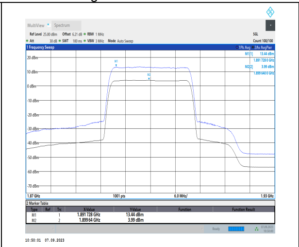
1-N2-PC3-15-20-H-2-CP-256QAM-Outer_Full-106@ 0-Ant2-9.45-100%-0.00-9.45-PASS-≤13
