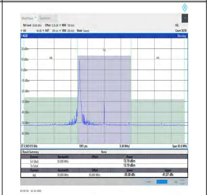
NTVN_N48_PC3_30_30_L_TID17_#1_-30_30
