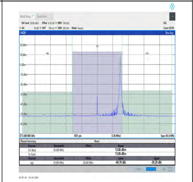
NTVN_N48_PC3_30_30_H_TID18_#1_-30_30
