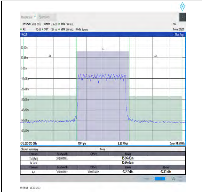
NTVN_N48_PC3_30_30_L_TID1_#1_-30_30
