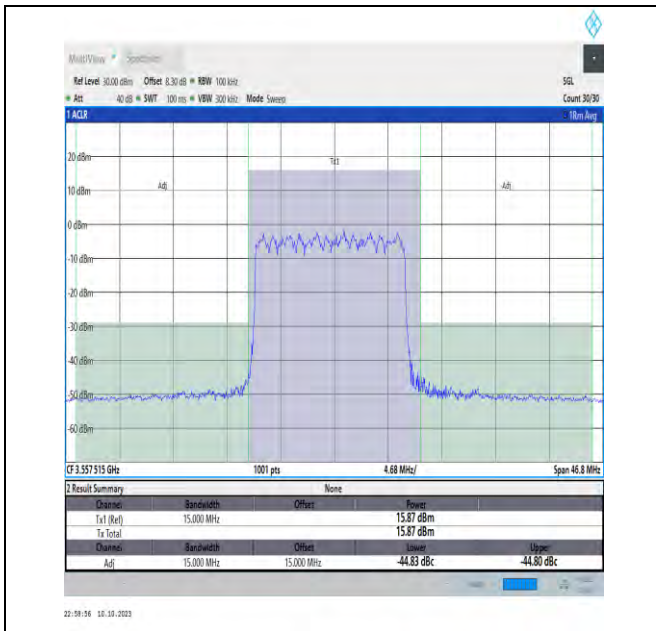
NTVN_N48_PC3_30_15_L_TID1_#1_-15_15
