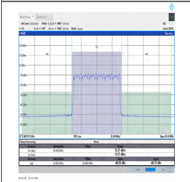
NTVN_N48_PC3_30_30_L_TID16_#1_-30_30
