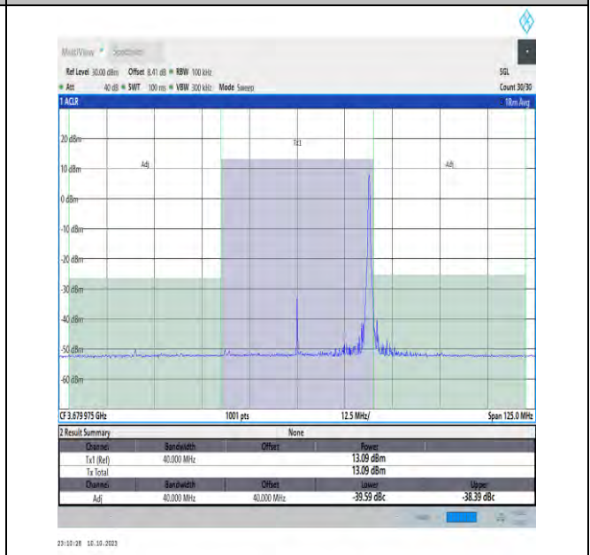
NTVN_N48_PC3_30_40_H_TID18_#1_-40_40
