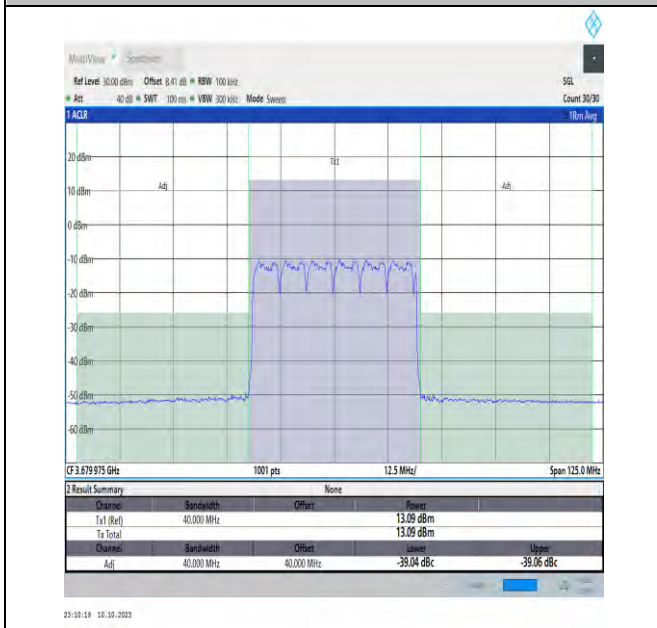
NTVN_N48_PC3_30_40_H_TID16_#1_-40_40
