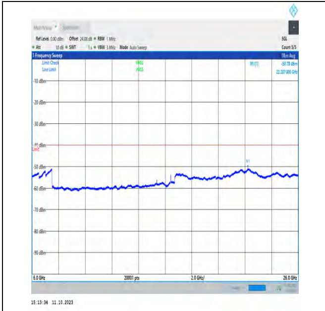
NTVN_N48_PC3_30_40_M_TID1_NS_01_6000_26000_#
