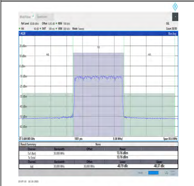
NTVN_N48_PC3_30_30_H_TID16_#1_-30_30
