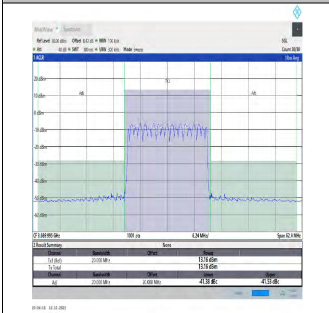
NTVN_N48_PC3_30_20_H_TID16_#1_-20_20
