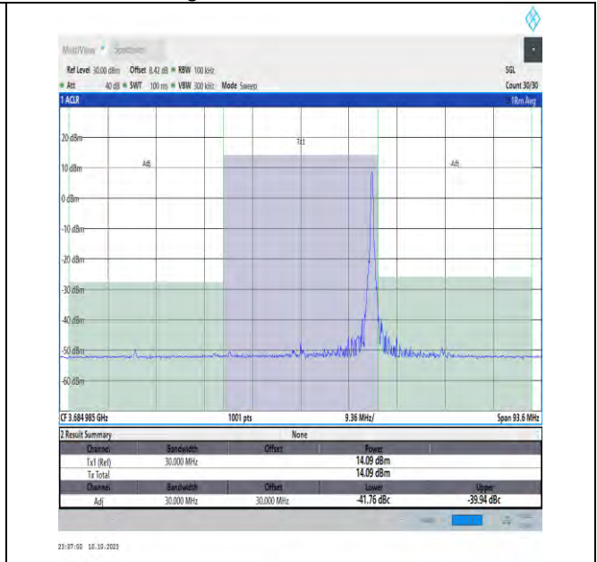
NTVN_N48_PC3_30_30_H_TID3_#1_-30_30
