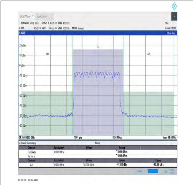
NTVN_N48_PC3_30_30_H_TID1_#1_-30_30
