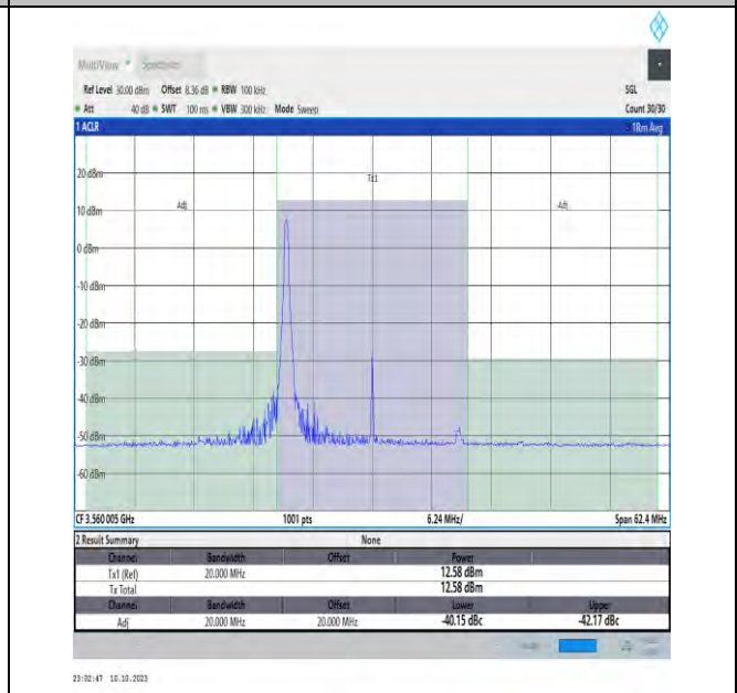
NTVN_N48_PC3_30_20_L_TID17_#1_-20_20
