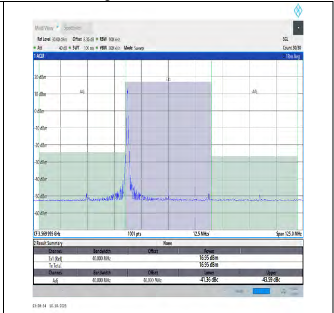
NTVN_N48_PC3_30_40_L_TID2_#1_-40_40
