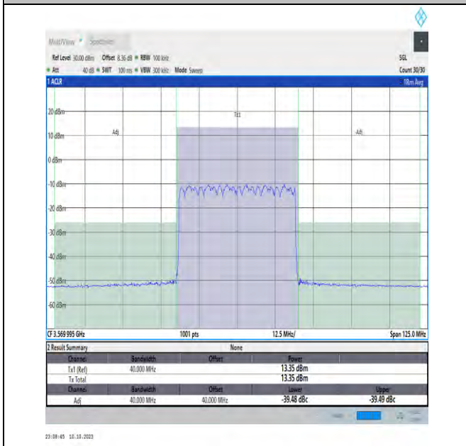
NTVN_N48_PC3_30_40_L_TID16_#1_-40_40
