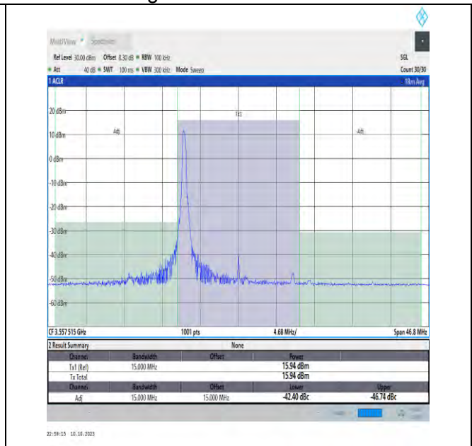
NTVN_N48_PC3_30_15_L_TID2_#1_-15_15
