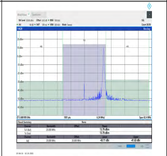
NTVN_N48_PC3_30_20_H_TID18_#1_-20_20
