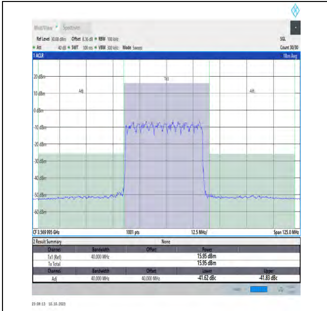
NTVN_N48_PC3_30_40_L_TID1_#1_-40_40
