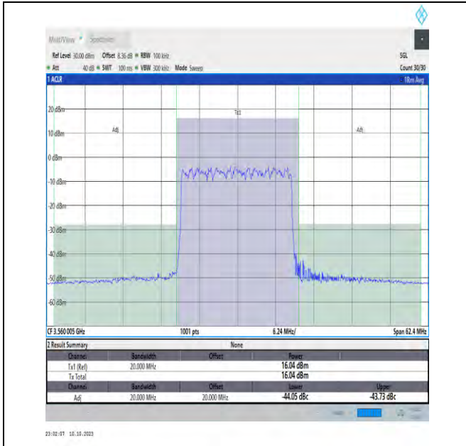
NTVN_N48_PC3_30_20_L_TID1_#1_-20_20
