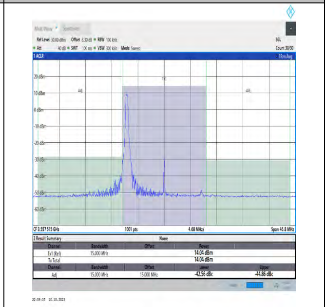
NTVN_N48_PC3_30_15_L_TID17_#1_-15_15
