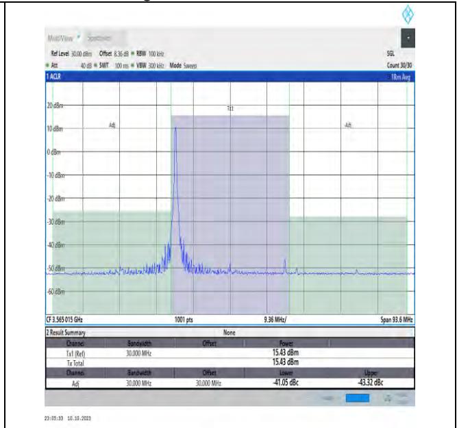
NTVN_N48_PC3_30_30_L_TID2_#1_-30_30
