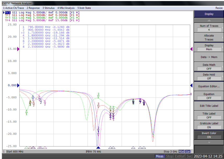
b.Div Antenna
