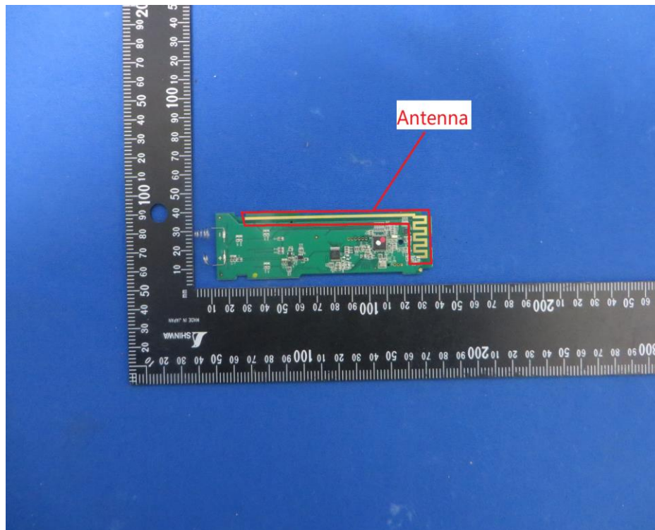
(3) EUT Photo
