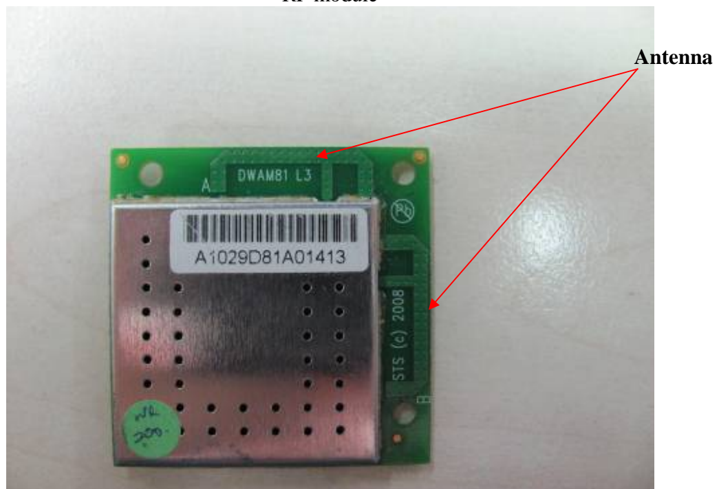
RF module
