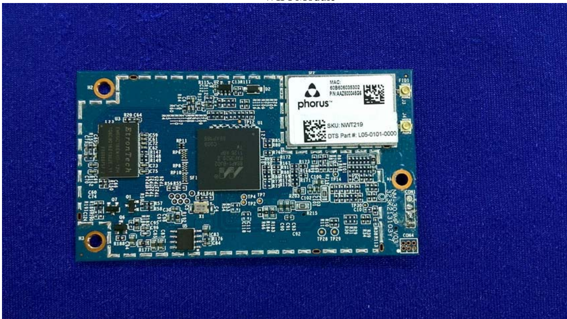
WIFI Module
