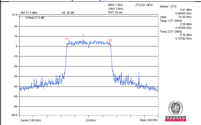
802.11ac (VHT80)_Chain 3 / CH138
