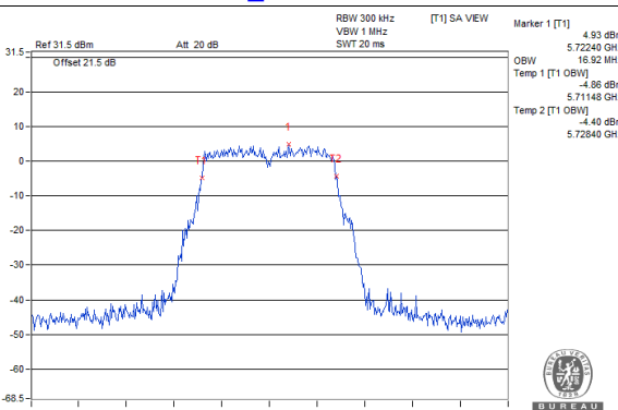
802.11a_Chain 2 / CH144
