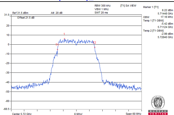
802.11ac (VHT20)_Chain 1 / CH144
