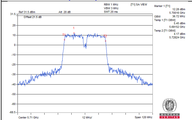
802.11ac (VHT40)_Chain 2 / CH142
