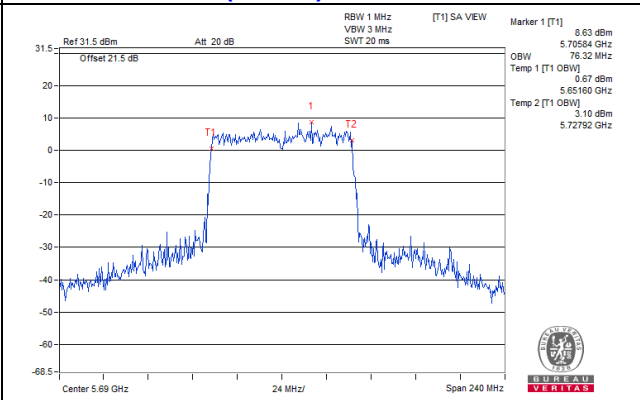
802.11ac (VHT80)_Chain 2 / CH138
