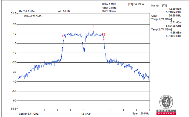
802.11ac (VHT40)_Chain 1 / CH142
