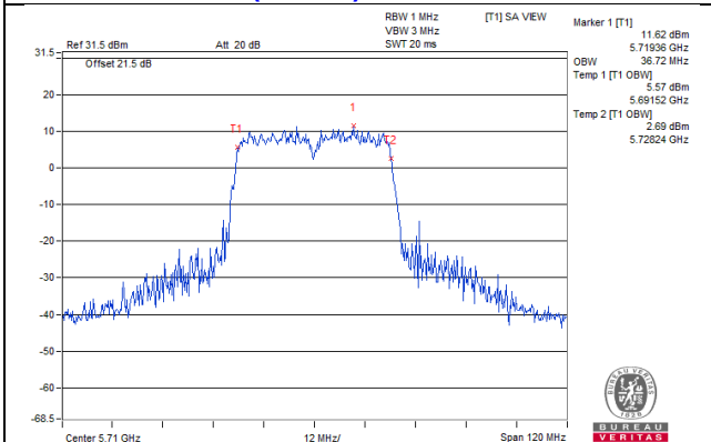
802.11ac (VHT40)_Chain 3 / CH142
