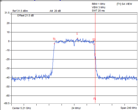
802.11ac(VHT80)_Chain2 / CH42
