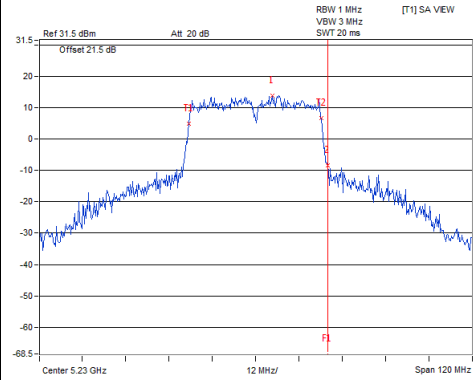
802.11ac(VHT40)_Chain2 / CH46
