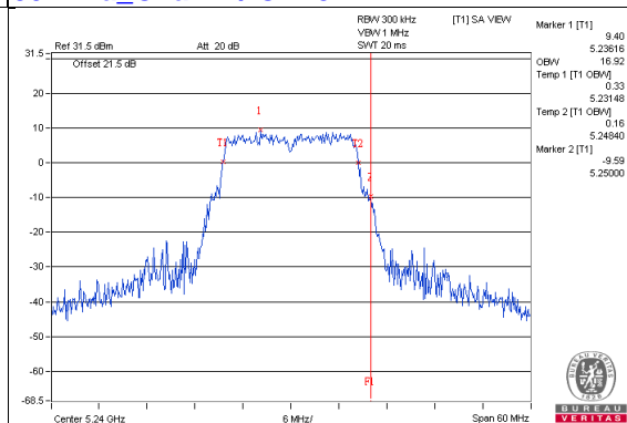
802.11a_Chain3 / CH48
