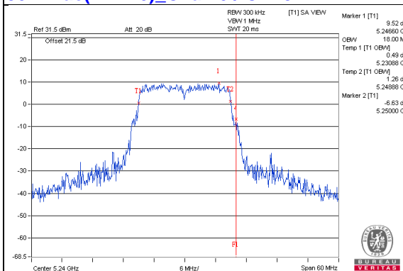
802.11ac(VHT20)_Chain2 / CH48
