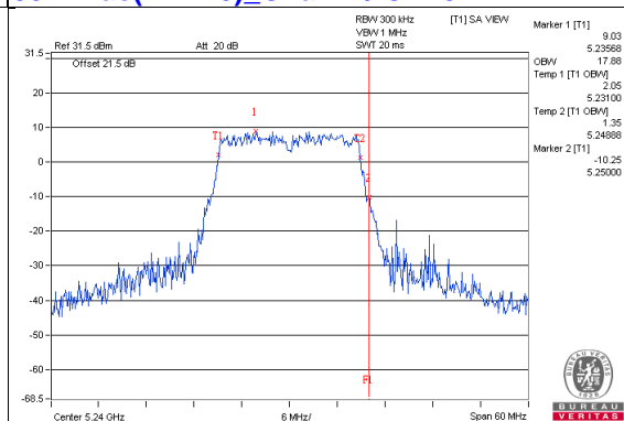
802.11ac(VHT20)_Chain3 / CH48
