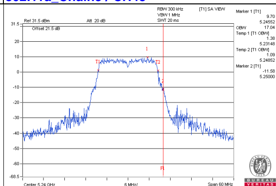
802.11ac(VHT20)_Chain1 / CH48
