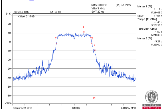
802.11a_Chain2 / CH48
