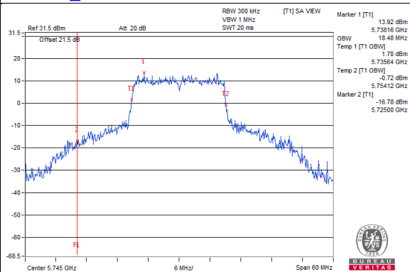
802.11a_Chain1 / CH149
