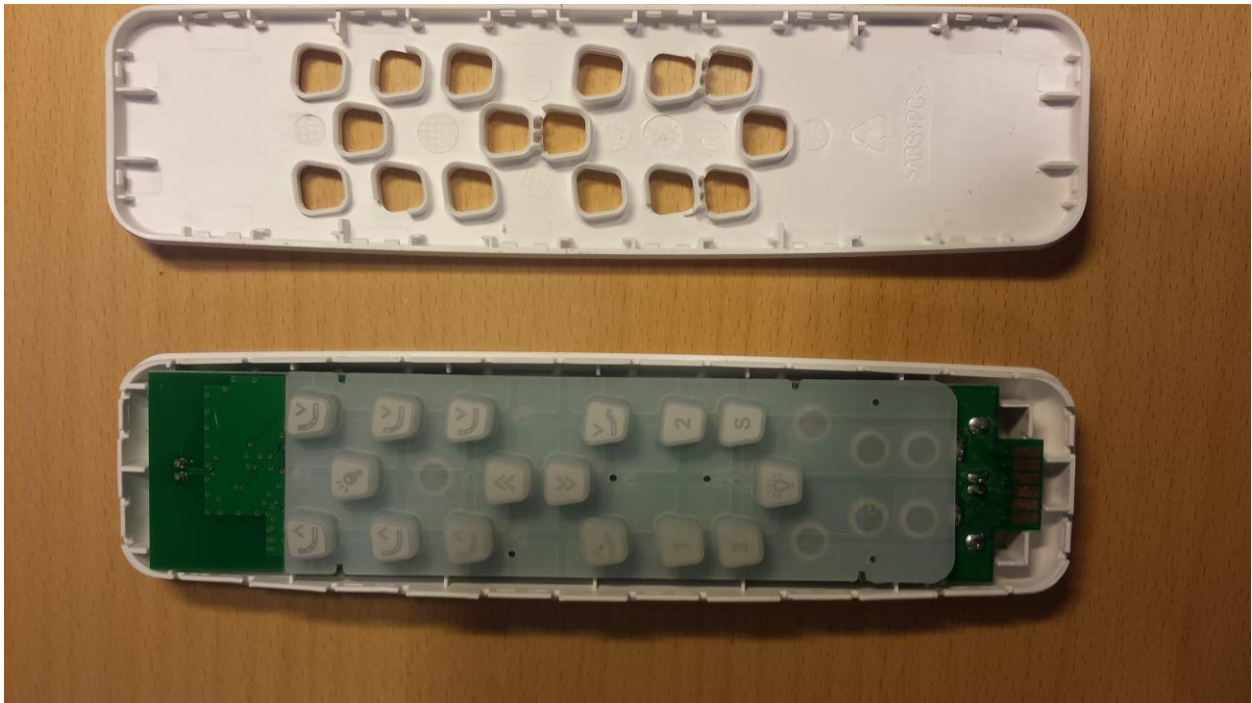
HC20
