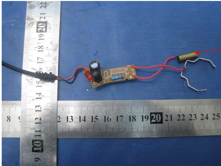
PCB-Front View(1)
