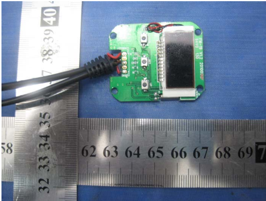
PCB-Front View(2)
