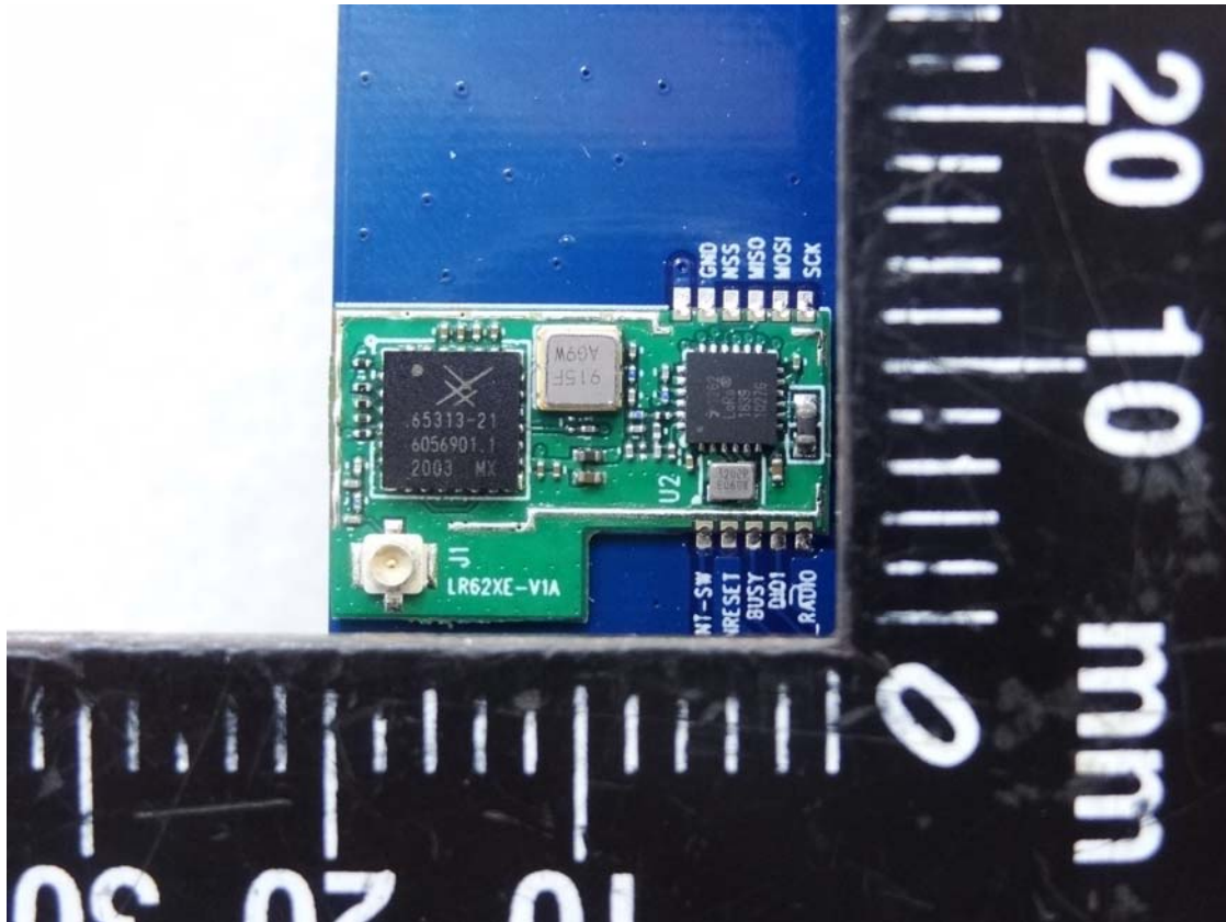
EUT-4. Antenna 1
