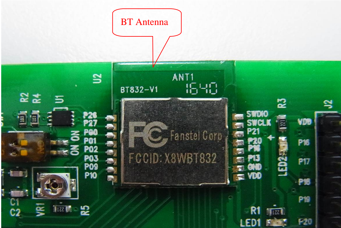
EUT 1 Model: BT832
