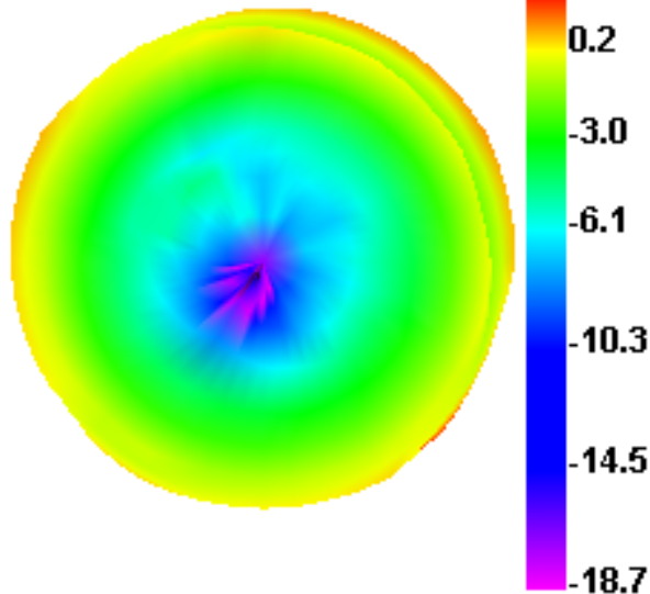
2450.000MHz E1
