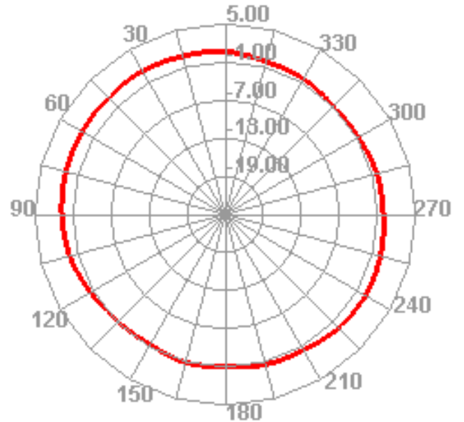
2450.000MHz H
