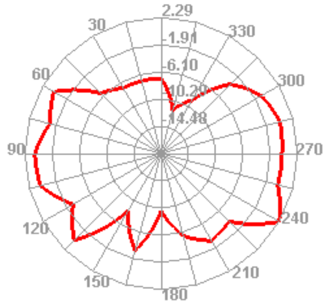
2450.000MHz E2
