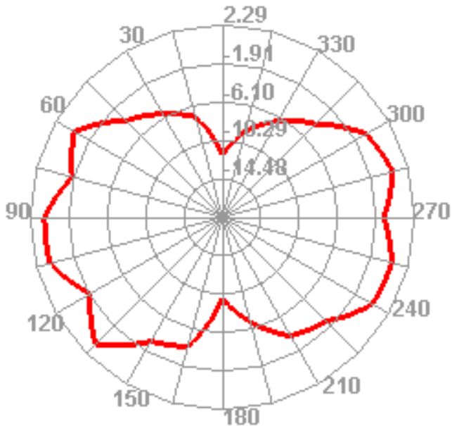
2450.000MHz E1
