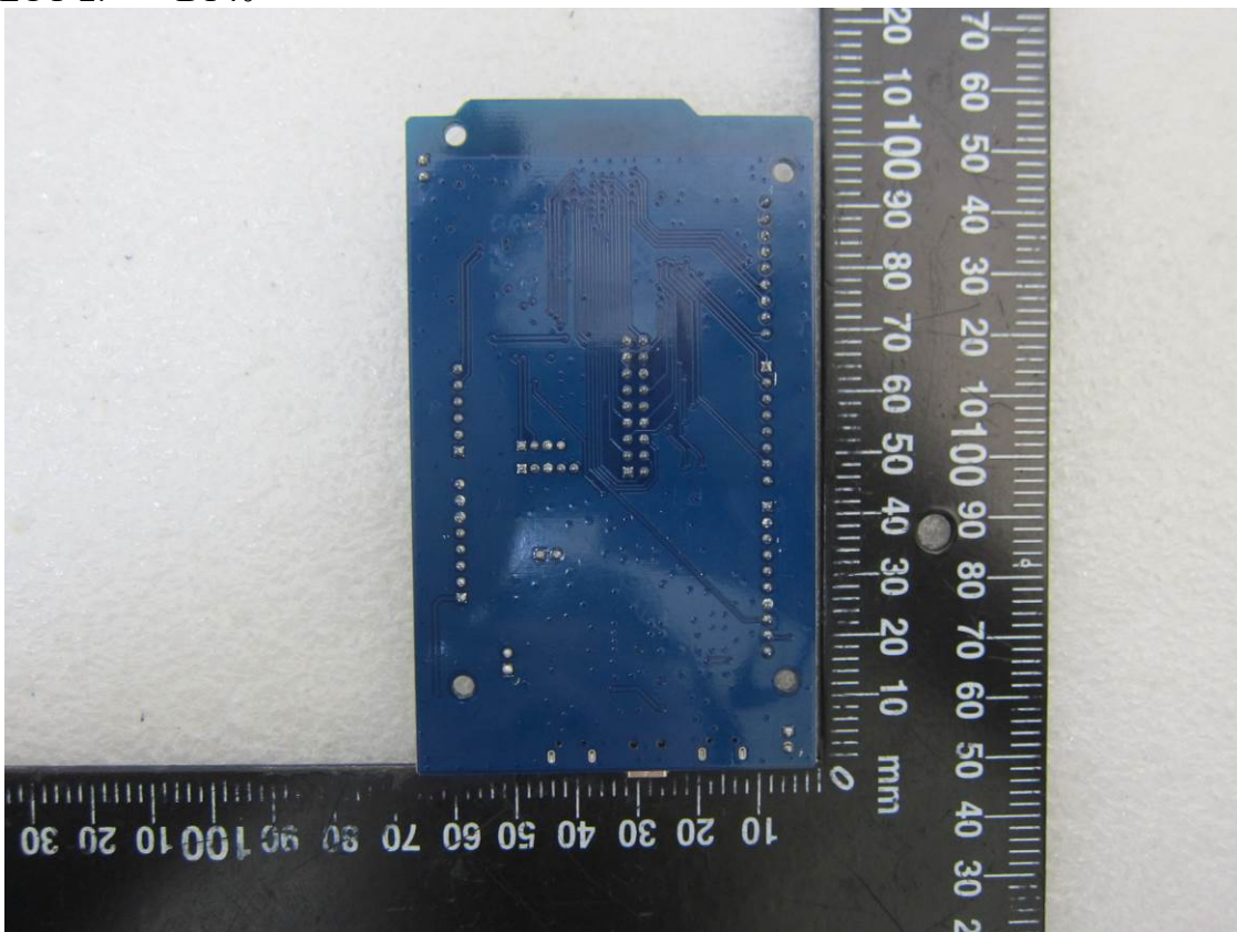
EUT-2. BT40
