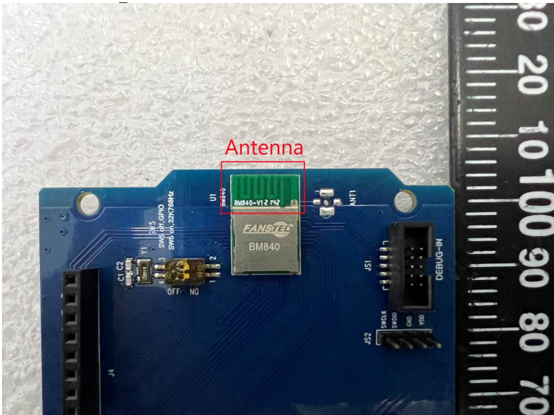
EUT-6. BM840_ANT
