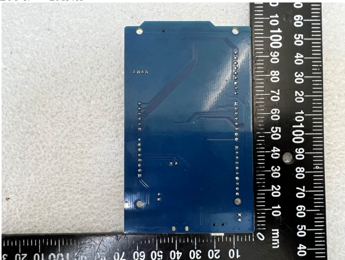
EUT-8. BM840P
