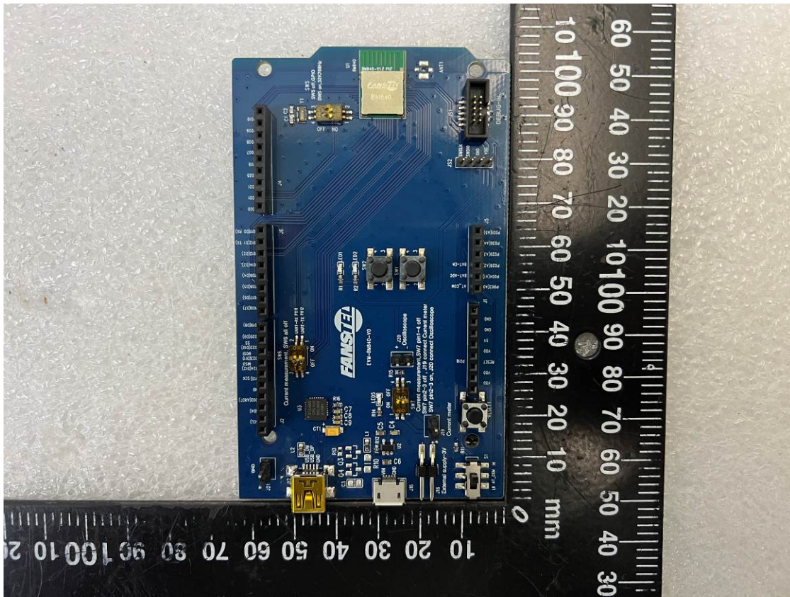
EUT-1. BM840
