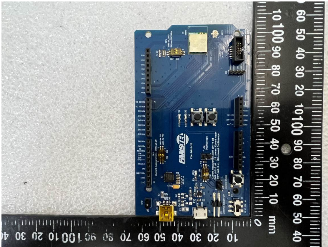
EUT-7. BM840P
