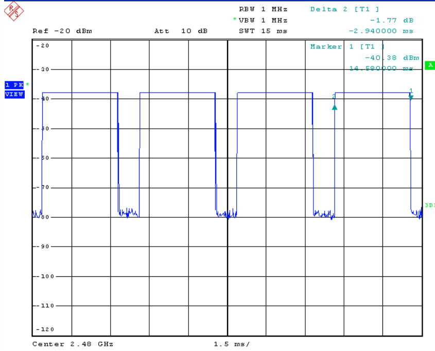
2480 MHz_DH5
