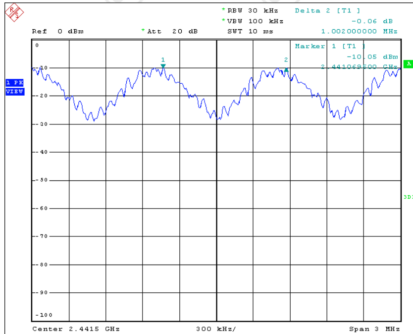
2441 MHz
