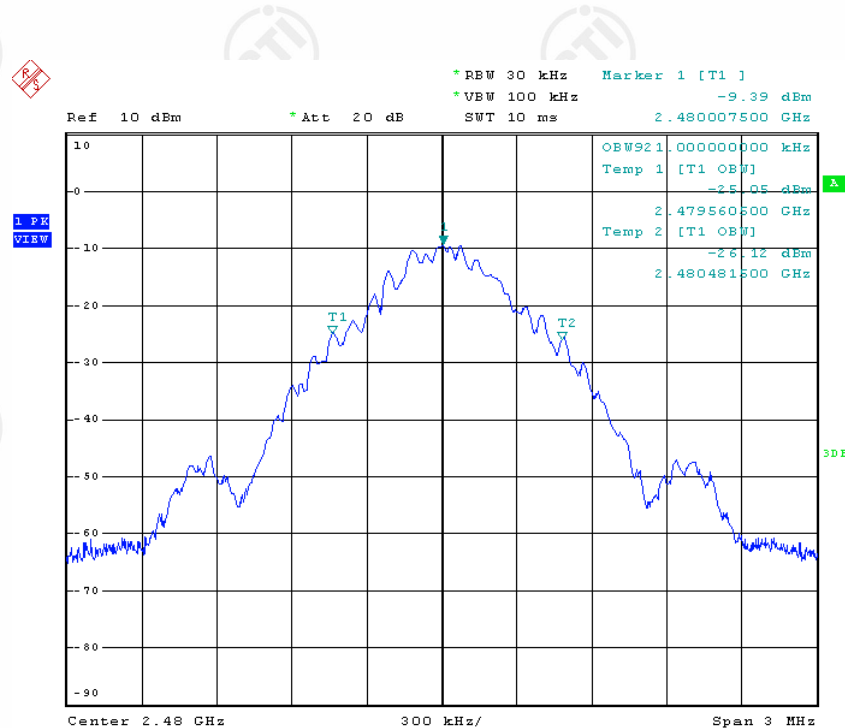
2480 MHz
