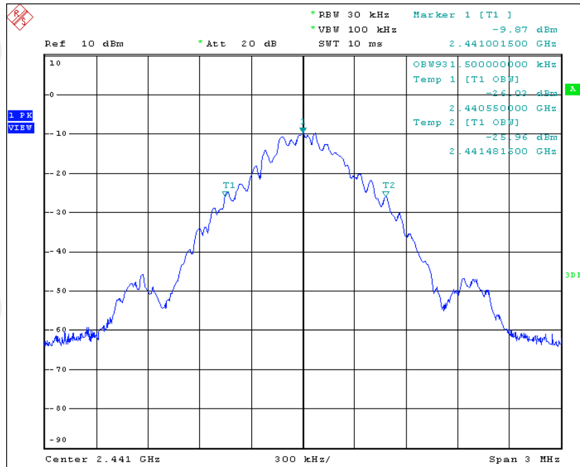
2441 MHz
