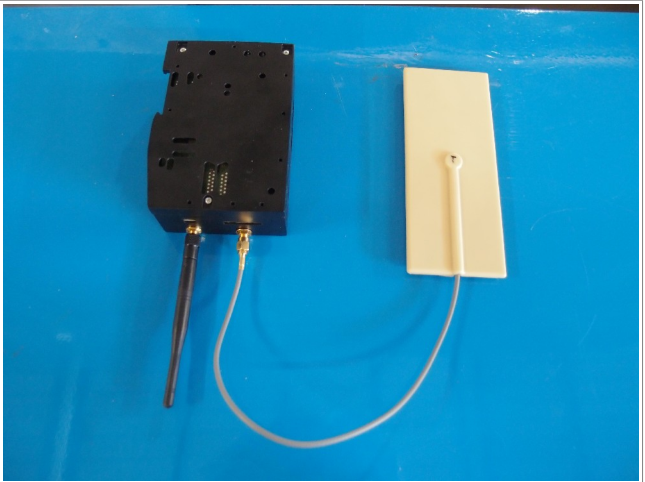
Top Side
