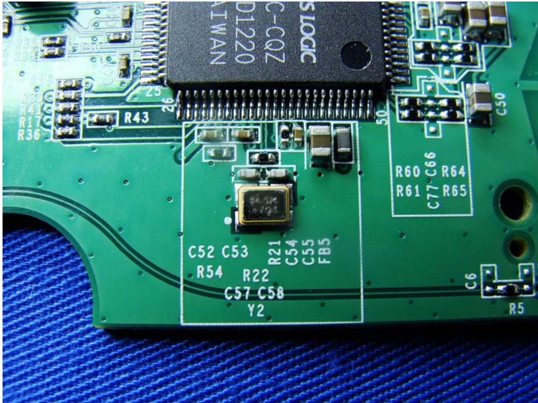
(10) EUT Photo (RF Chip)
