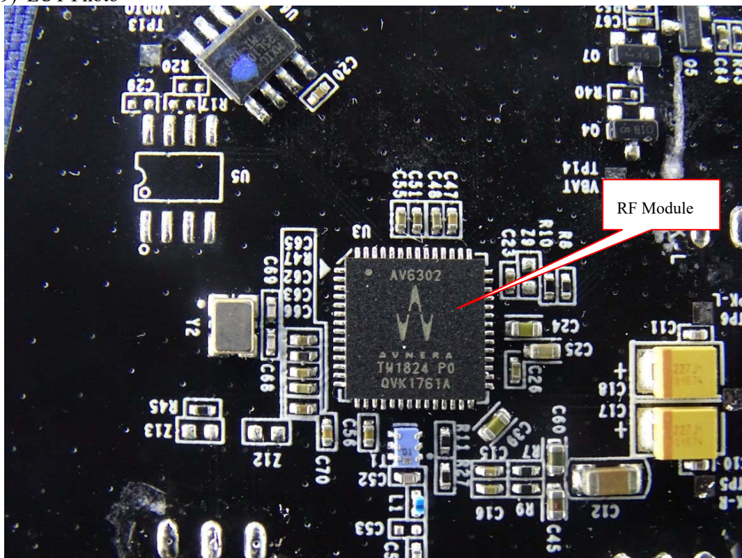
(10) EUT Photo
