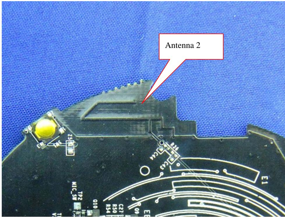
(19) EUT Photo
