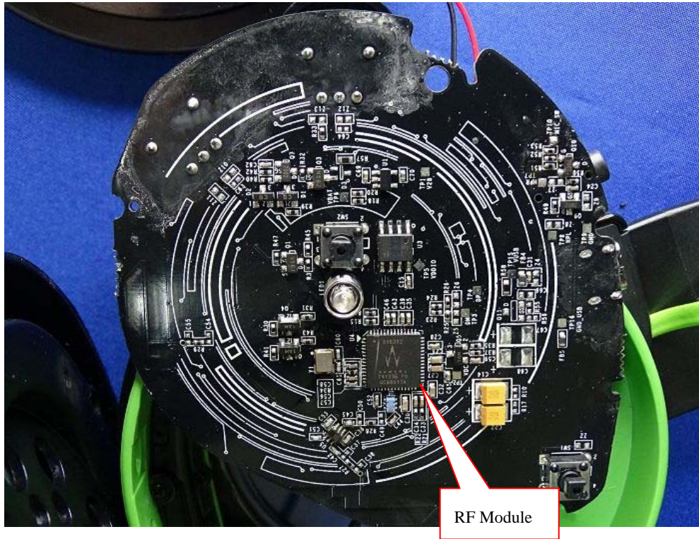
(9) EUT Photo
