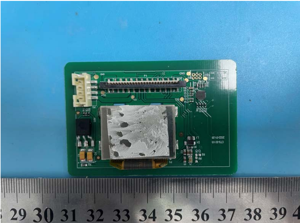
Antenna-BT,BLE,WIFI
