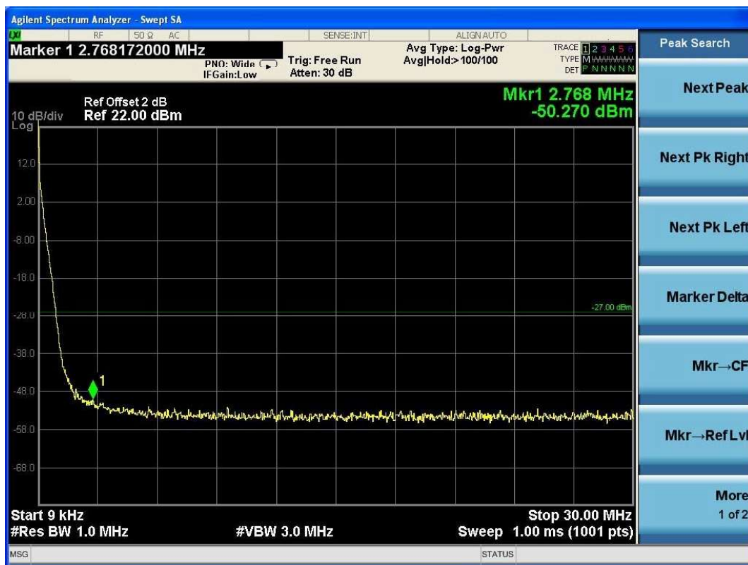
(Plot 4.9.3 B2: Channel 157: 5785MHz @ 802.11a)
