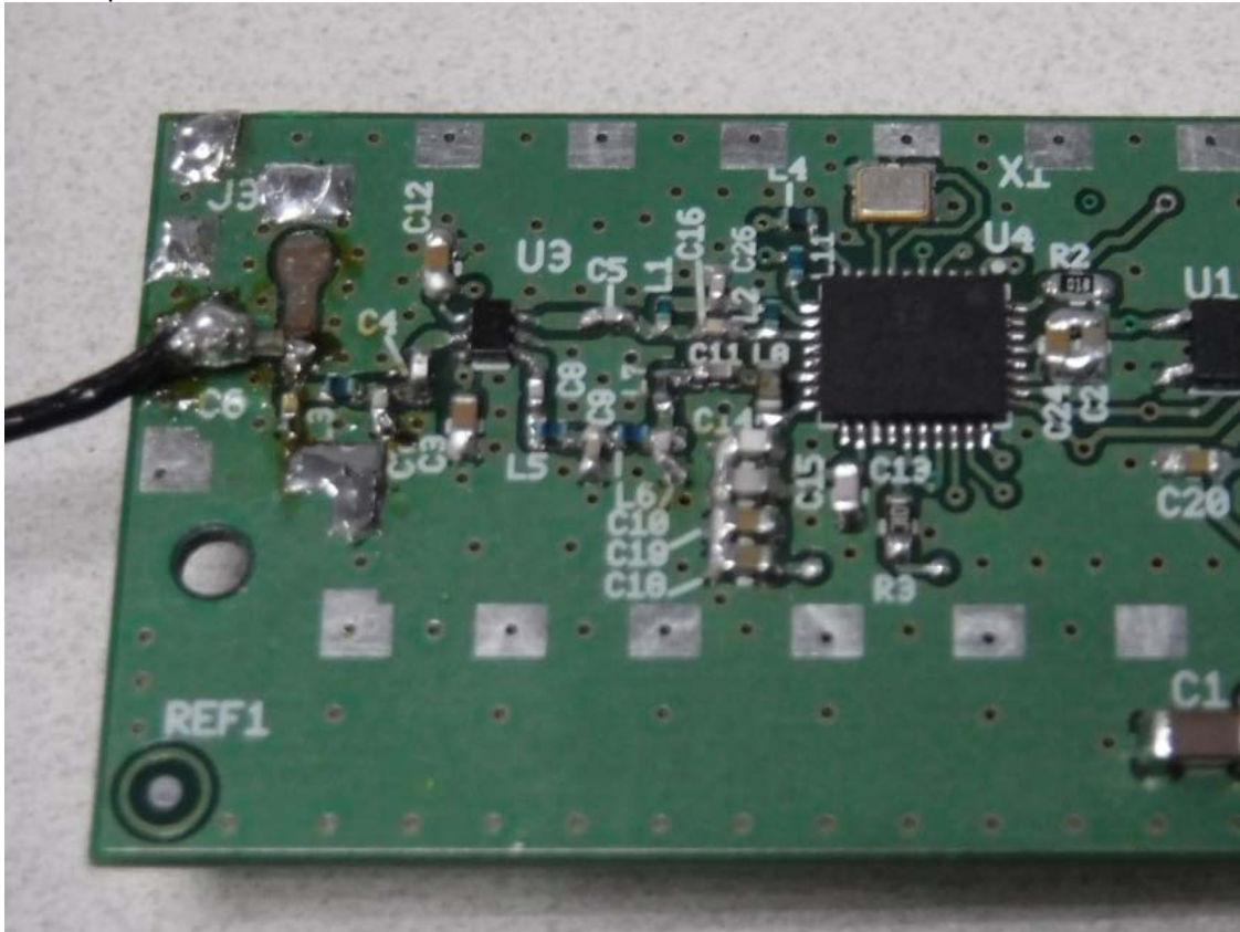
PCB Top
