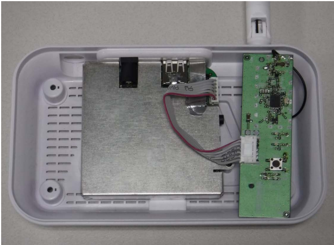
PCB Top
