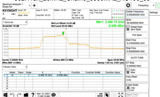
802.11ax_20MHz_Chain0_5500MHz_RU26_0
