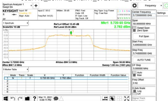
802.11a_20MHz_Chain1_5720MHz_UNII 2C
