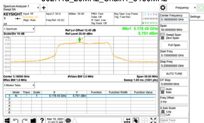
802.11a_20MHz_Chain1_5180MHz
