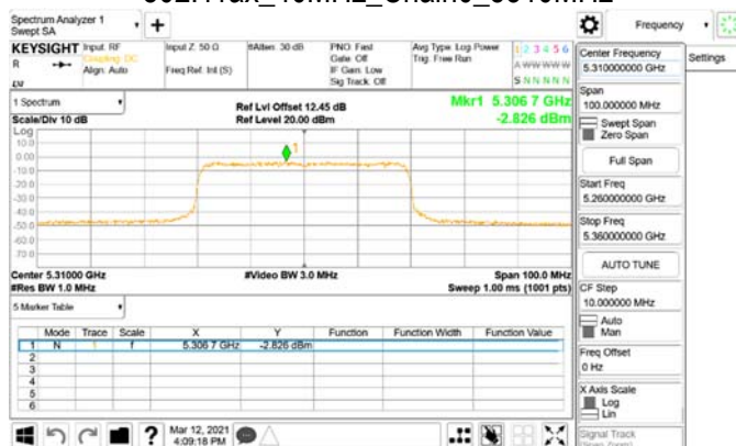
802.11ax_40MHz_Chain0_5310MHz_RU242_62
