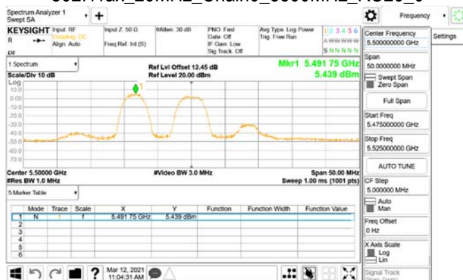
802.11ax_20MHz_Chain0_5500MHz_RU52_37
