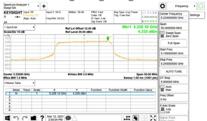
802.11n_20MHz_Chain0_5220MHz
