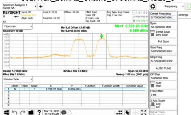
802.11ax_20MHz_Chain0_5700MHz_RU52_40
