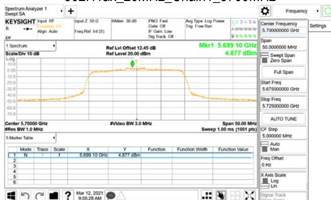
802.11ax_20MHz_Chain1_5700MHz_RU106_54
