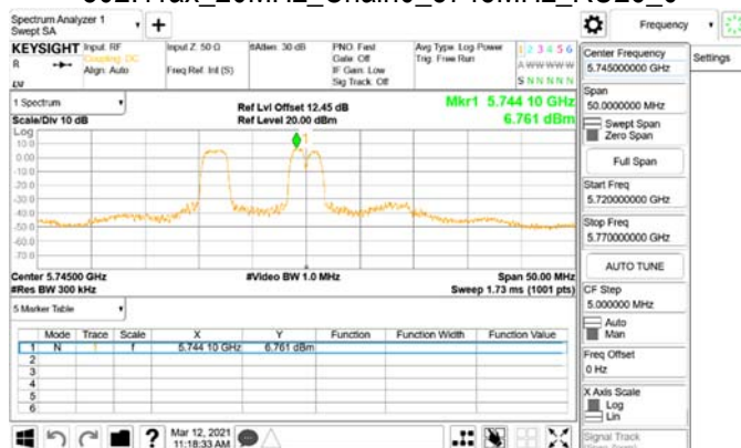
802.11ax_20MHz_Chain0_5745MHz_RU52_37
