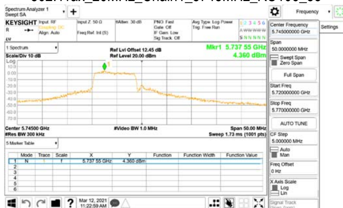
802.11ax_20MHz_Chain1_5745MHz_RU26_0
