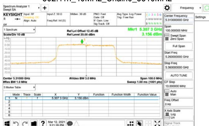
802.11n_40MHz_Chain0_5310MHz
