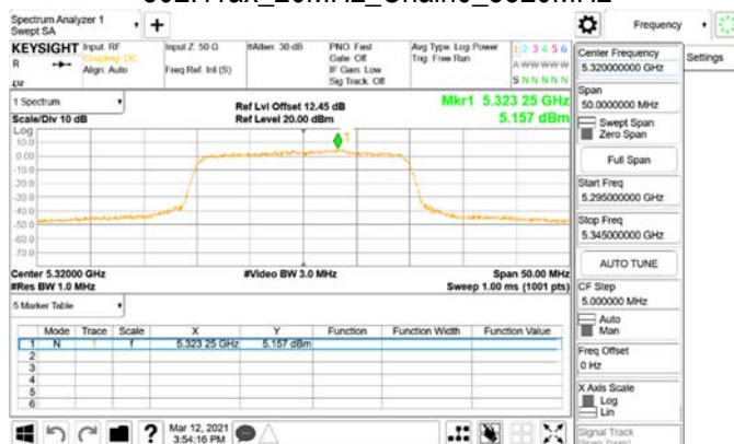
802.11ax_20MHz_Chain0_5320MHz_RU106_54
