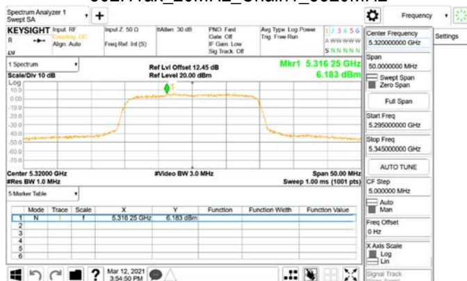
802.11ax_20MHz_Chain1_5320MHz_RU106_54
