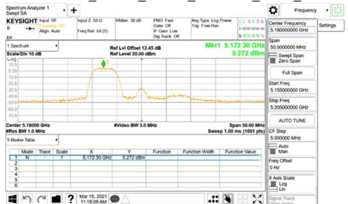
802.11ax_20MHz_Chain0_5180MHz_RU52_37
