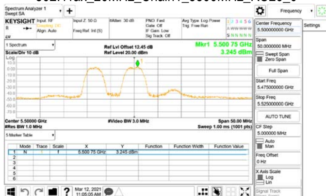
802.11ax_20MHz_Chain1_5500MHz_RU52_37
