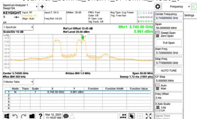
802.11ax_20MHz_Chain1_5745MHz_RU26_0
