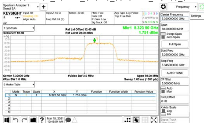
802.11ax_20MHz_Chain0_5320MHz_RU106_54
