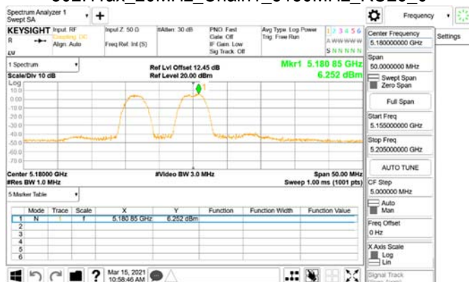
802.11ax_20MHz_Chain1_5180MHz_RU52_37
