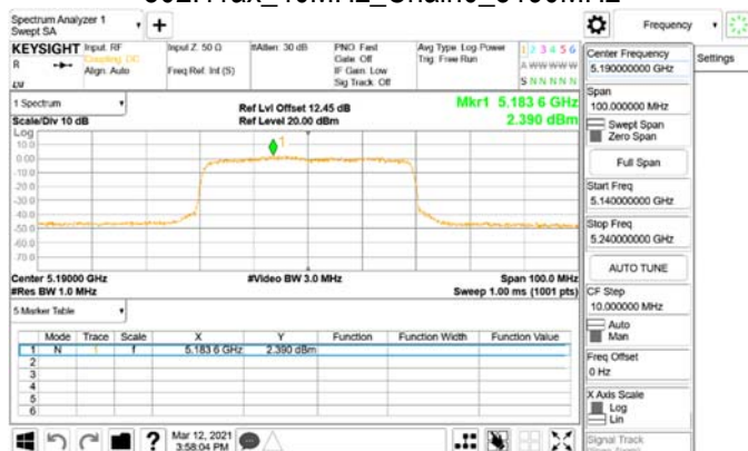
802.11ax_40MHz_Chain0_5190MHz_RU242_61
