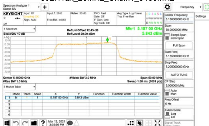
802.11ax_20MHz_Chain1_5180MHz_RU106_53
